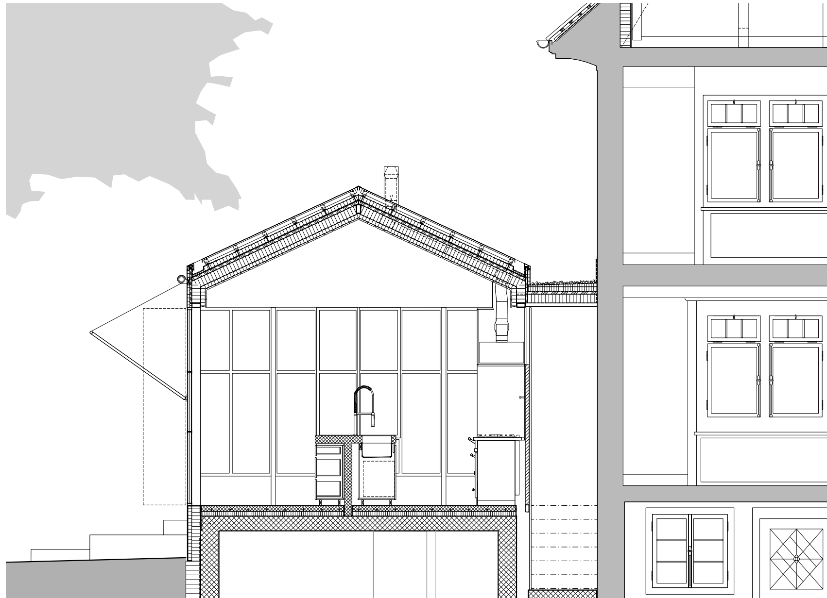
Schnitt DD
