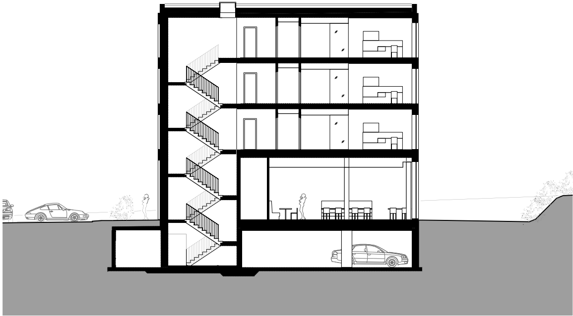
Coupe Est
