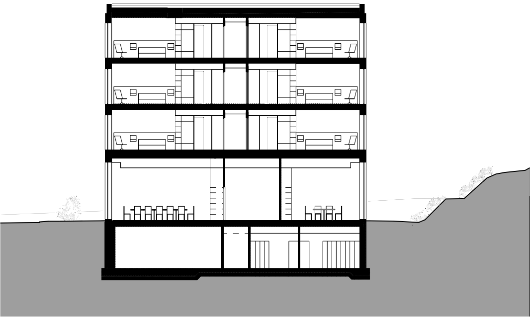
Coupe Ouest
