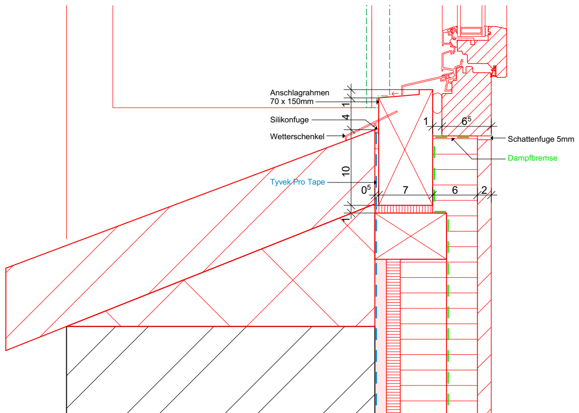
Detail Fenster OG 1:5
