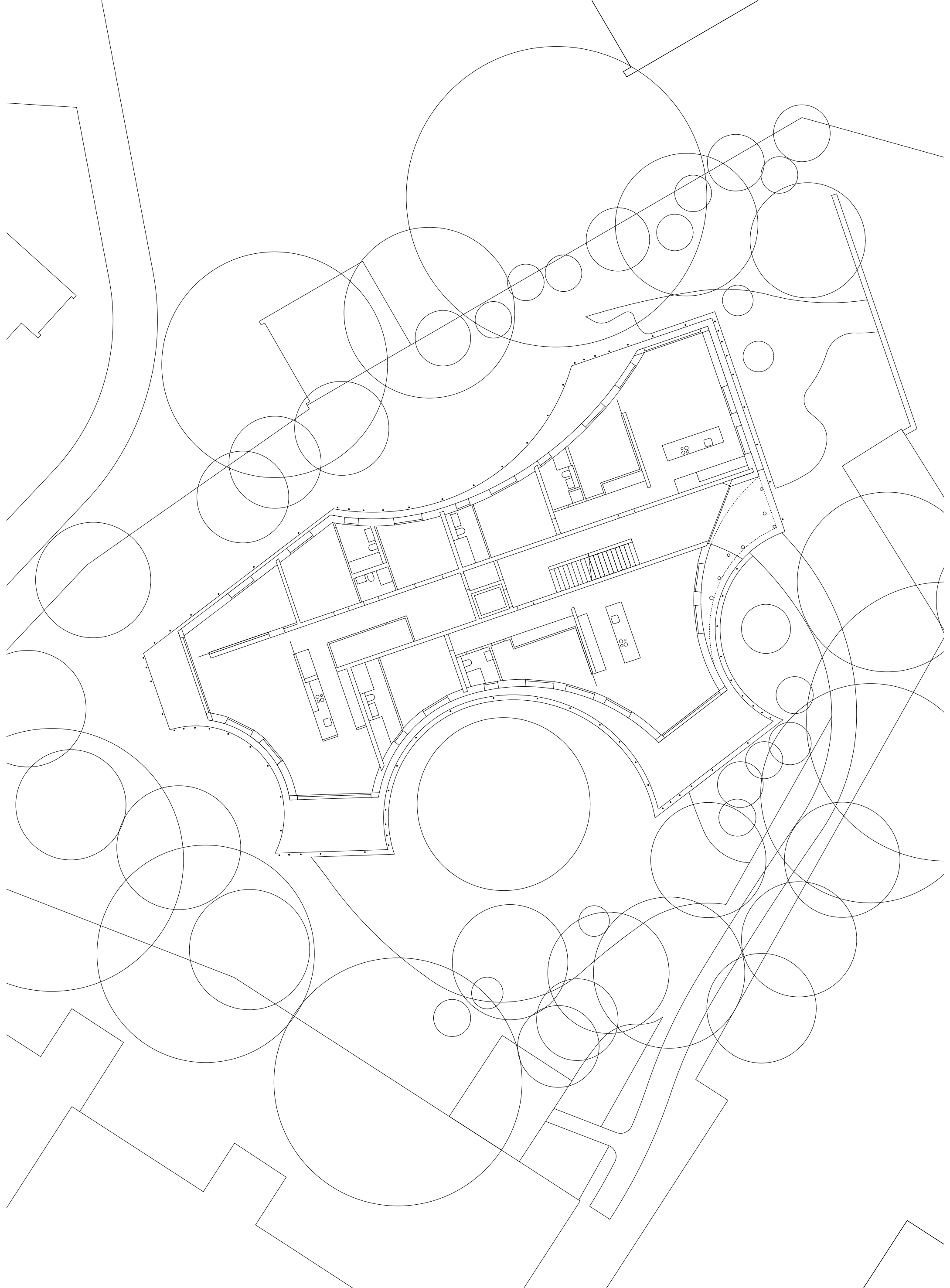
Erdgeschoss 1:200
