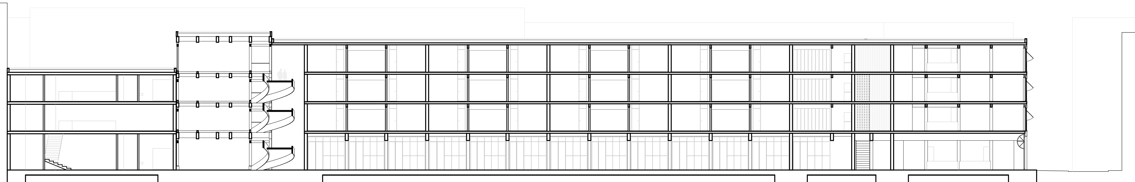
Längsschnitt_2 1:200
