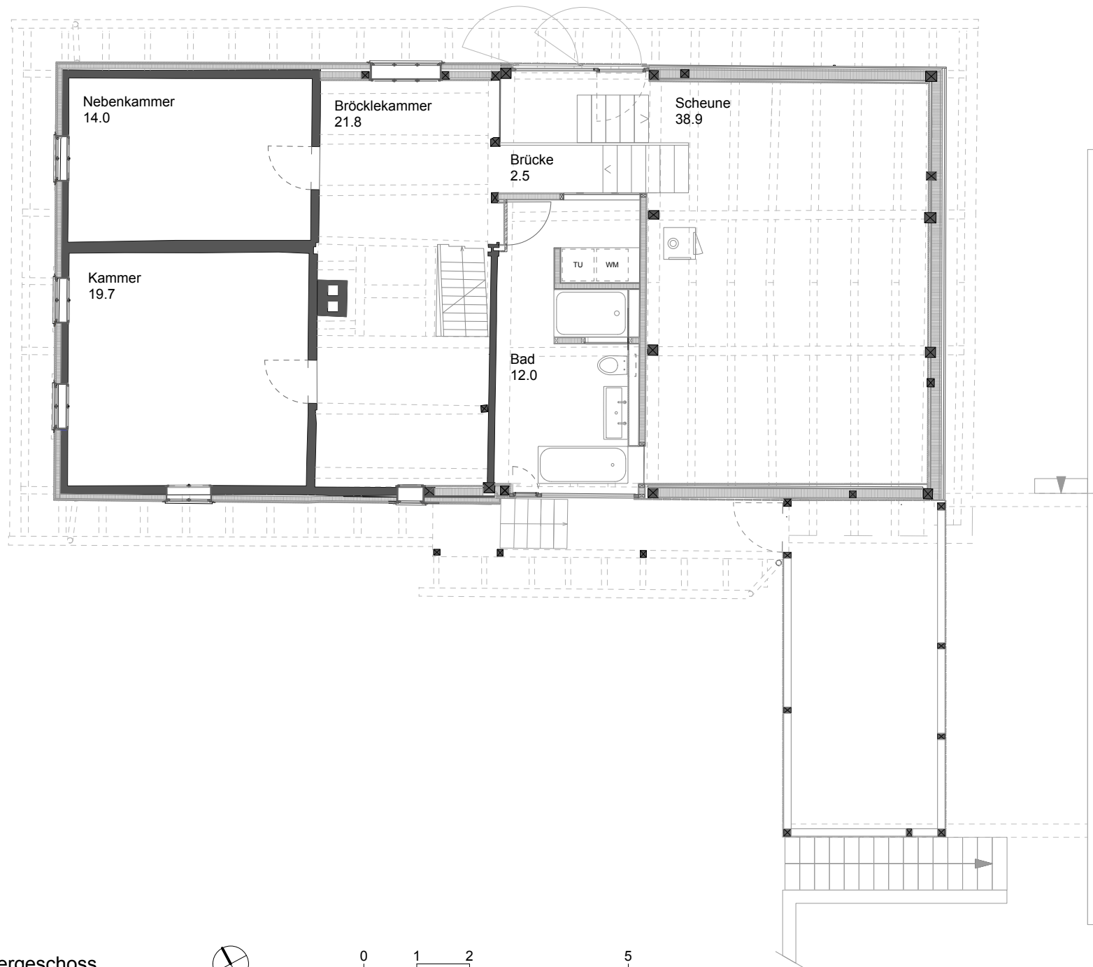
Grundriss Obergeschoss
