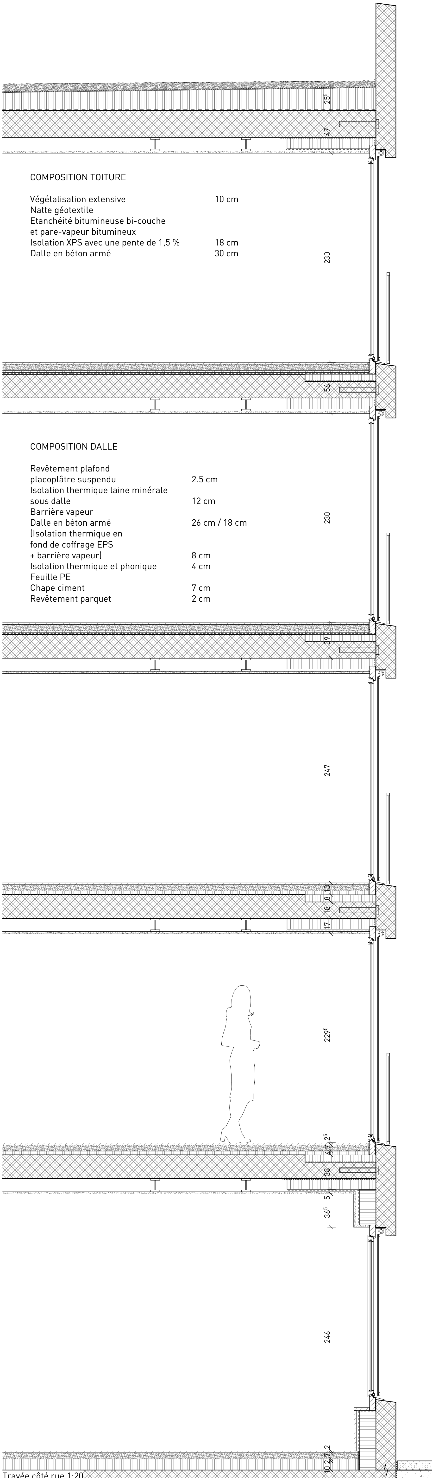
Travée côté rue 1:20
