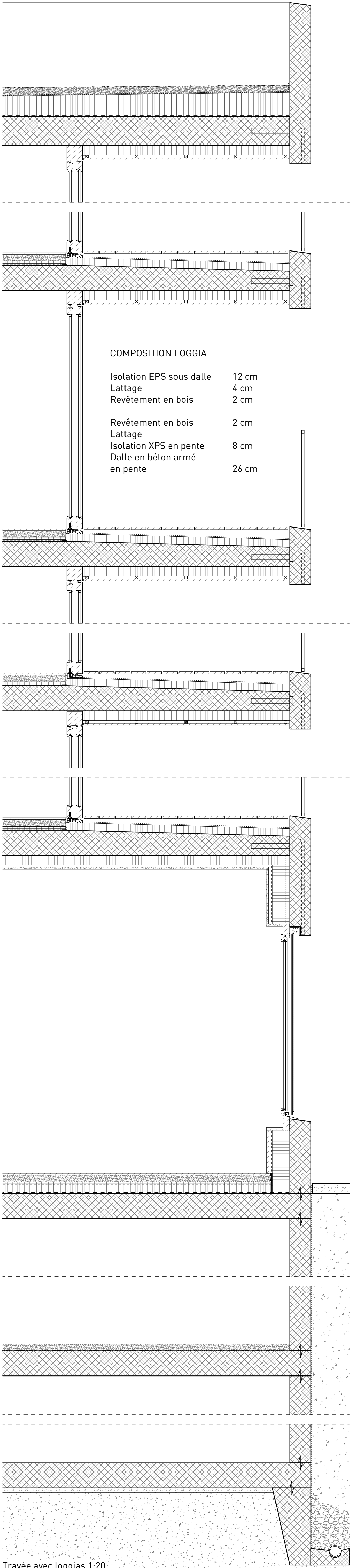
Travée avec loggias 1:20
