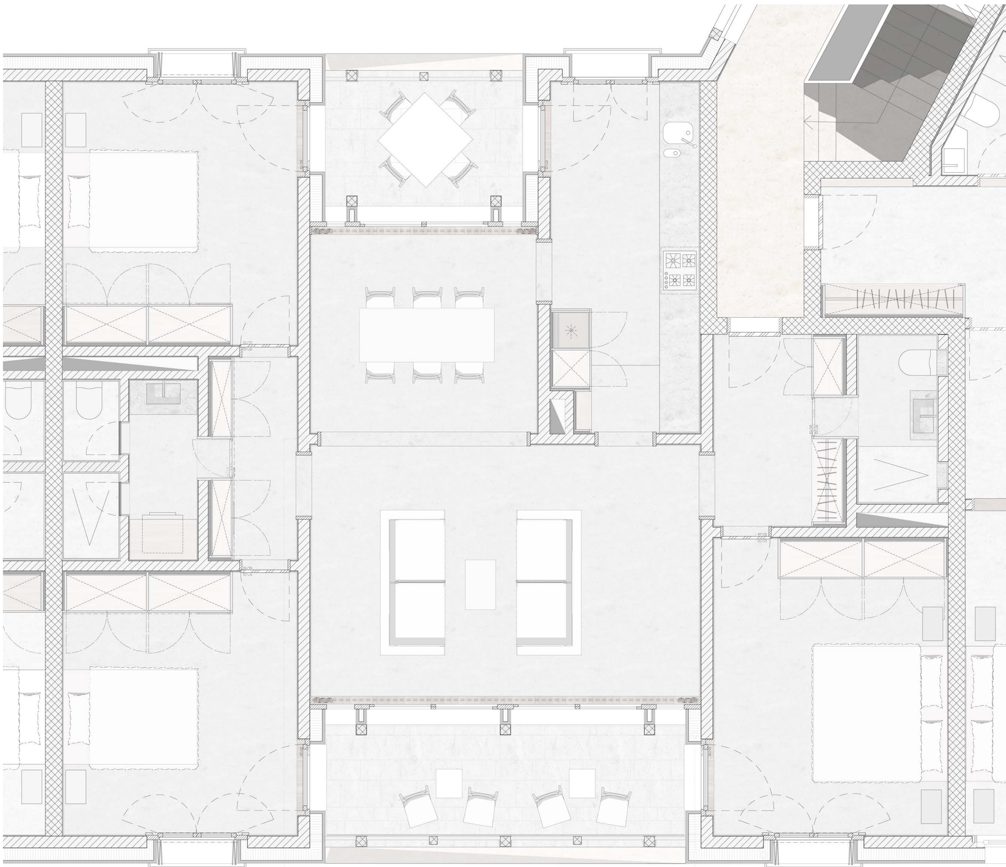
grundriss 1:33
