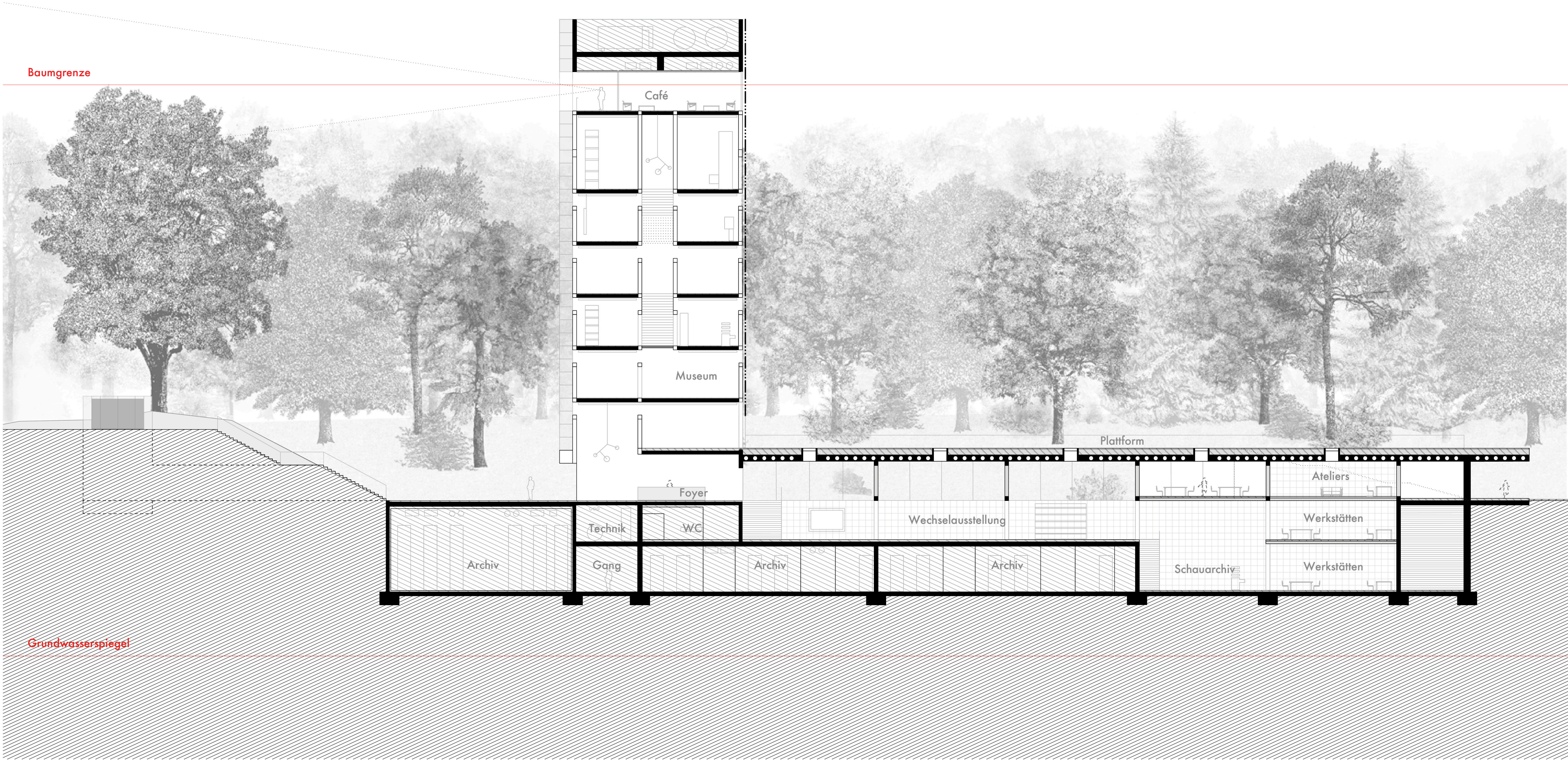
Schnitt bb
