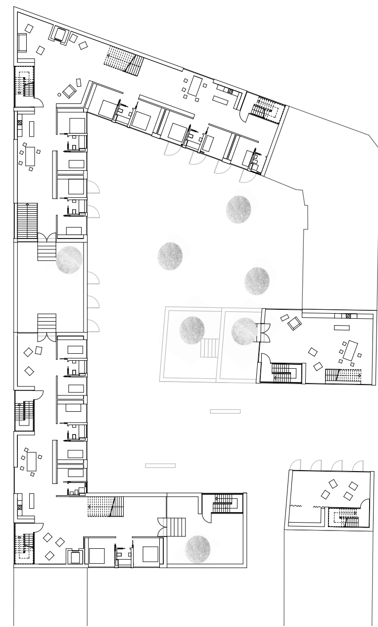
3. OG M_1:500
