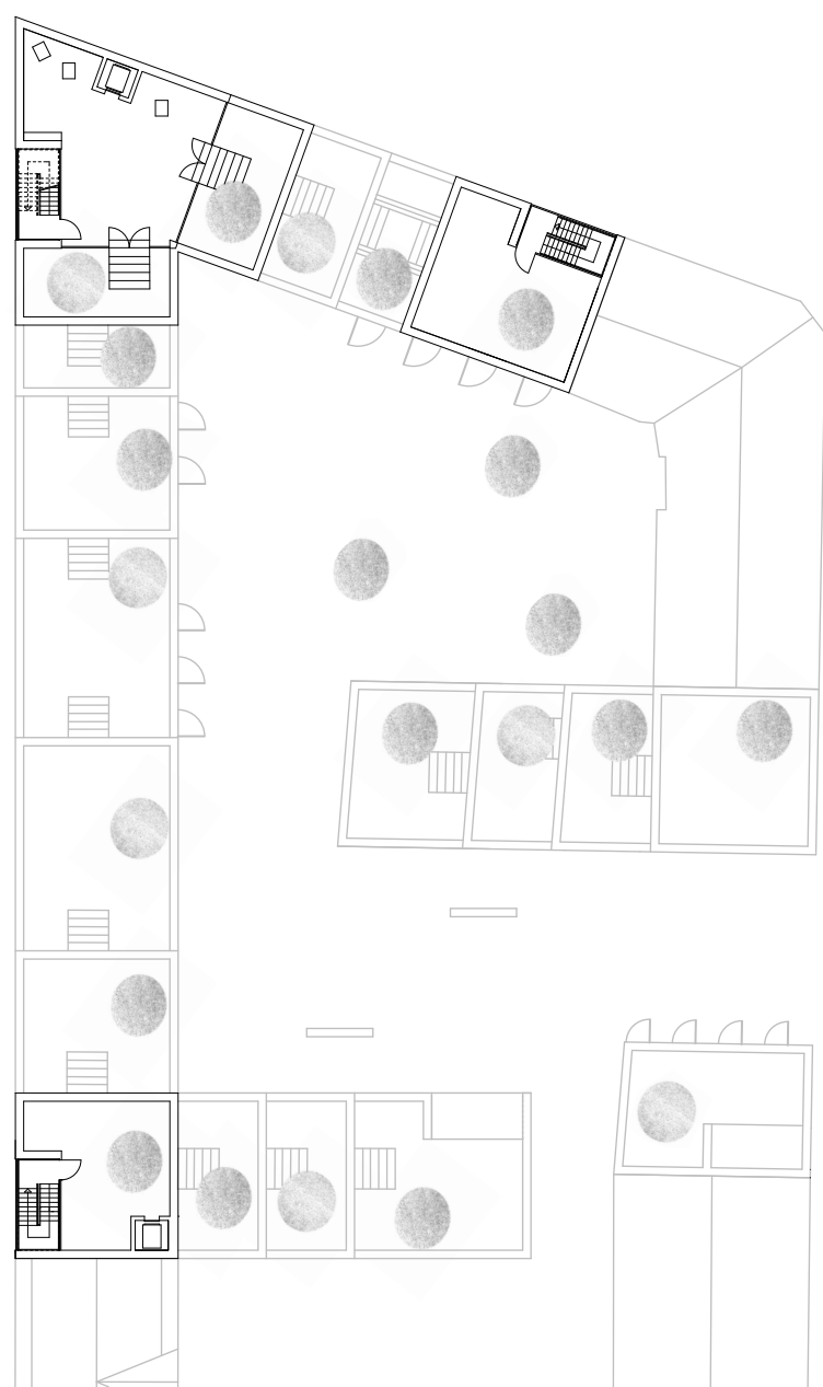
6. OG M_1:500
