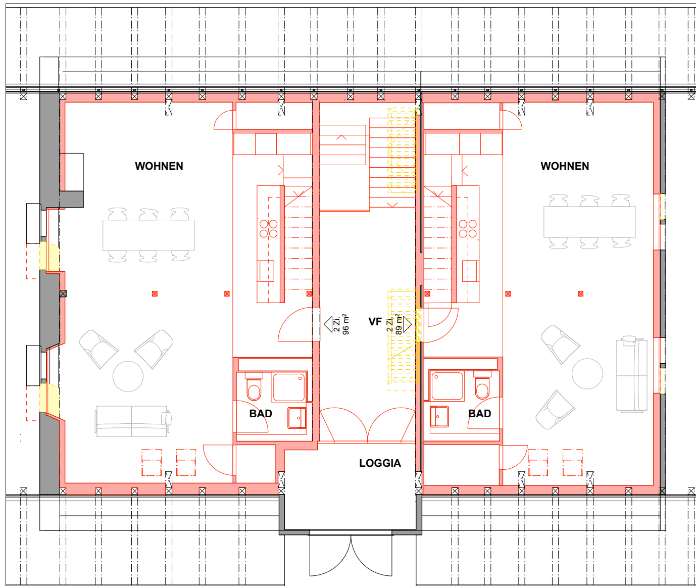
1. Dachgeschoss 1:100
