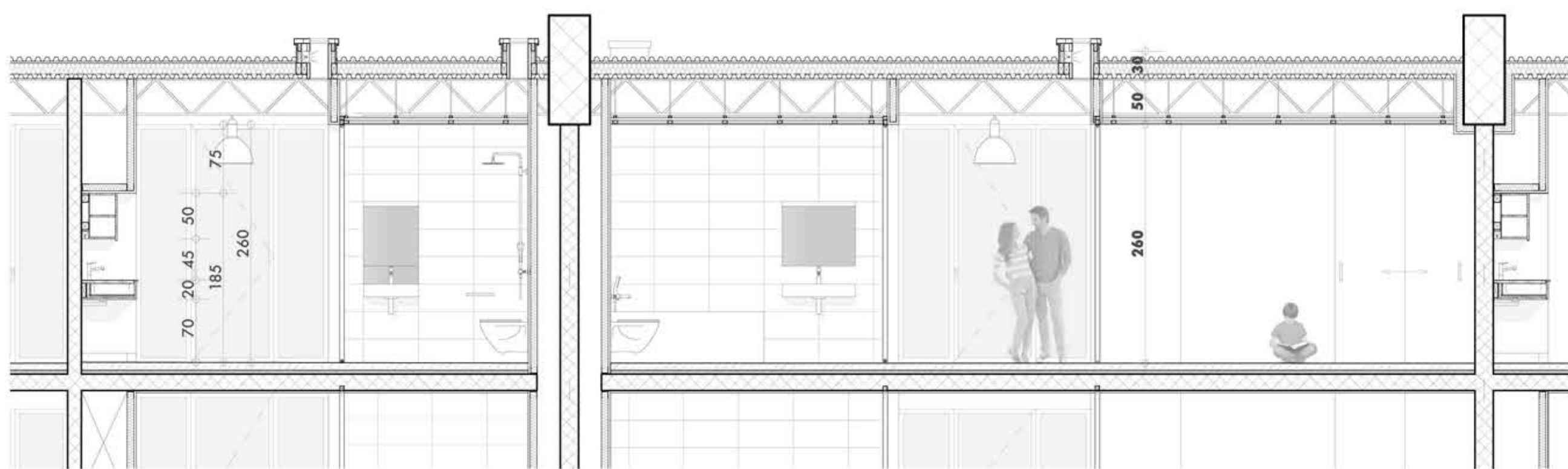
COUPE AA
