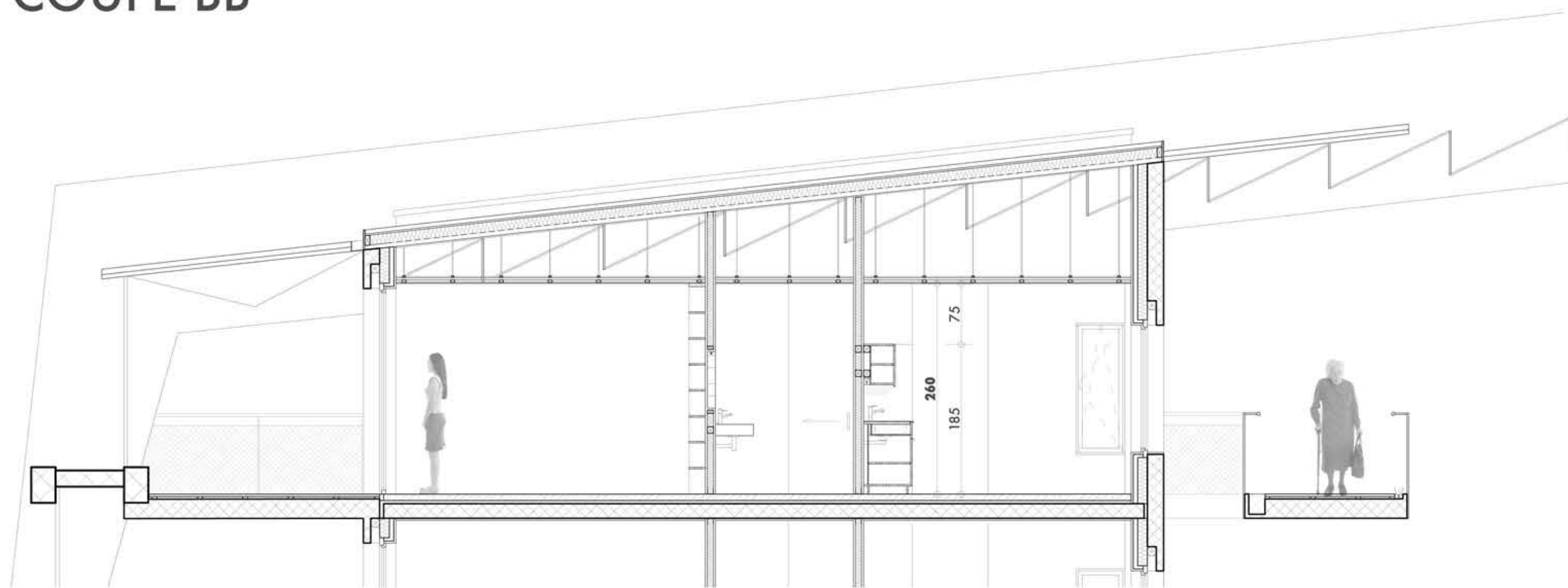
COUPE CC
