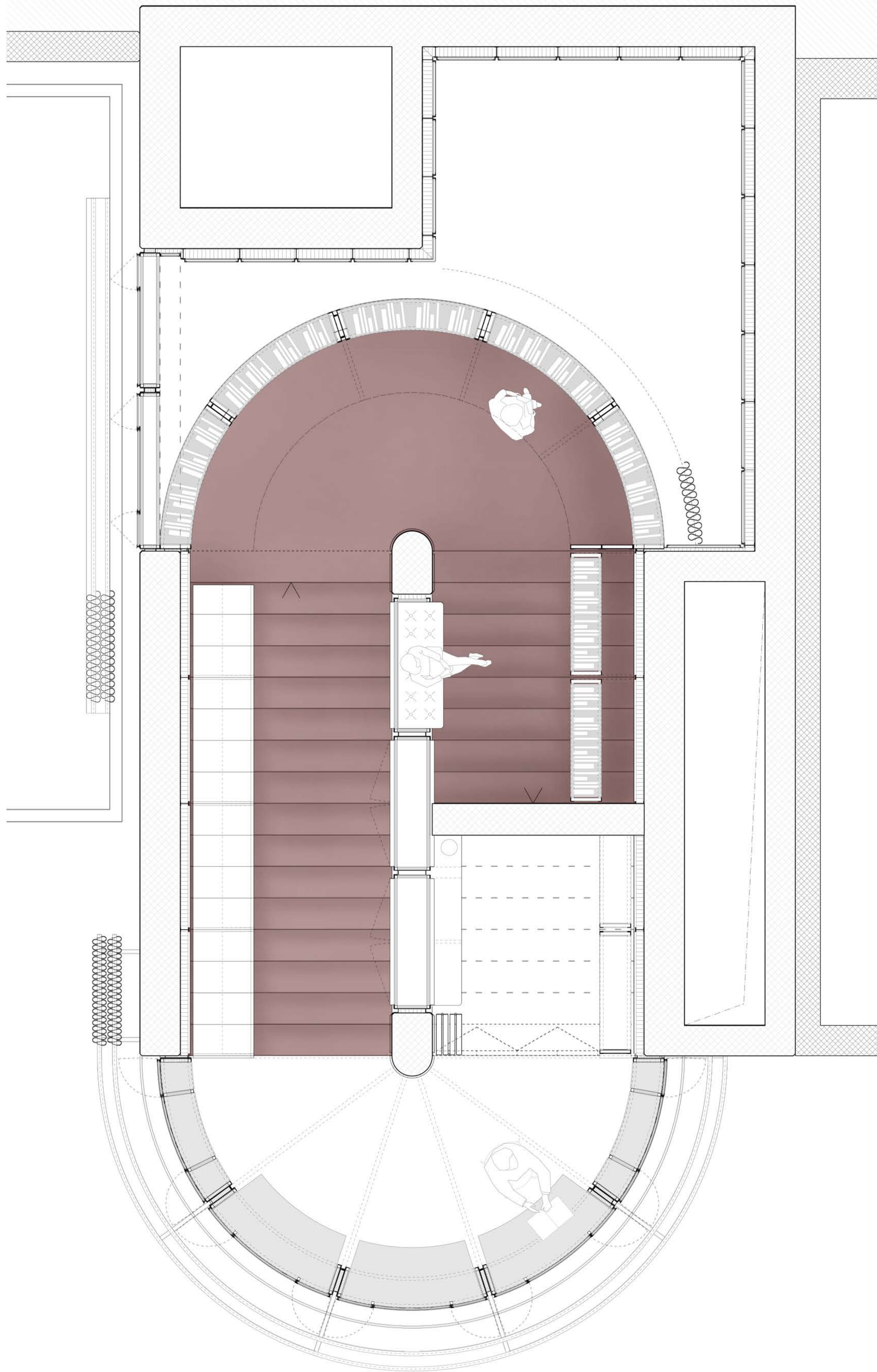
_Podest 1 1:20
