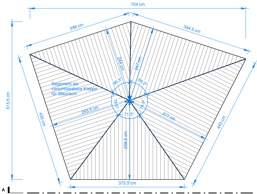
Grundriss 1 : 50
