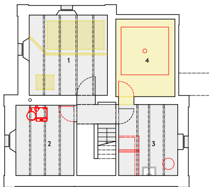
Kellergeschoss
