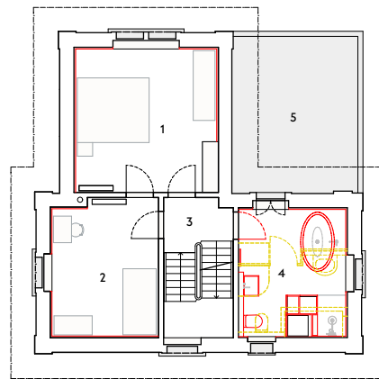
Obergeschoss
