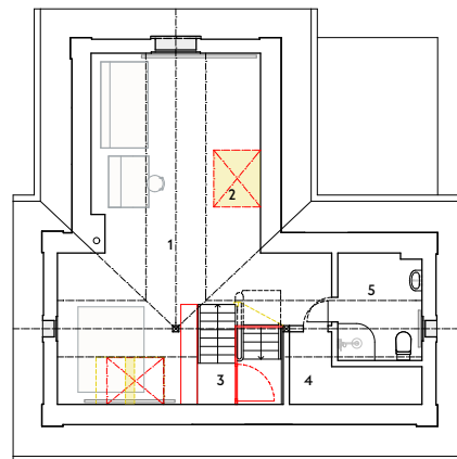
Dachgeschoss
