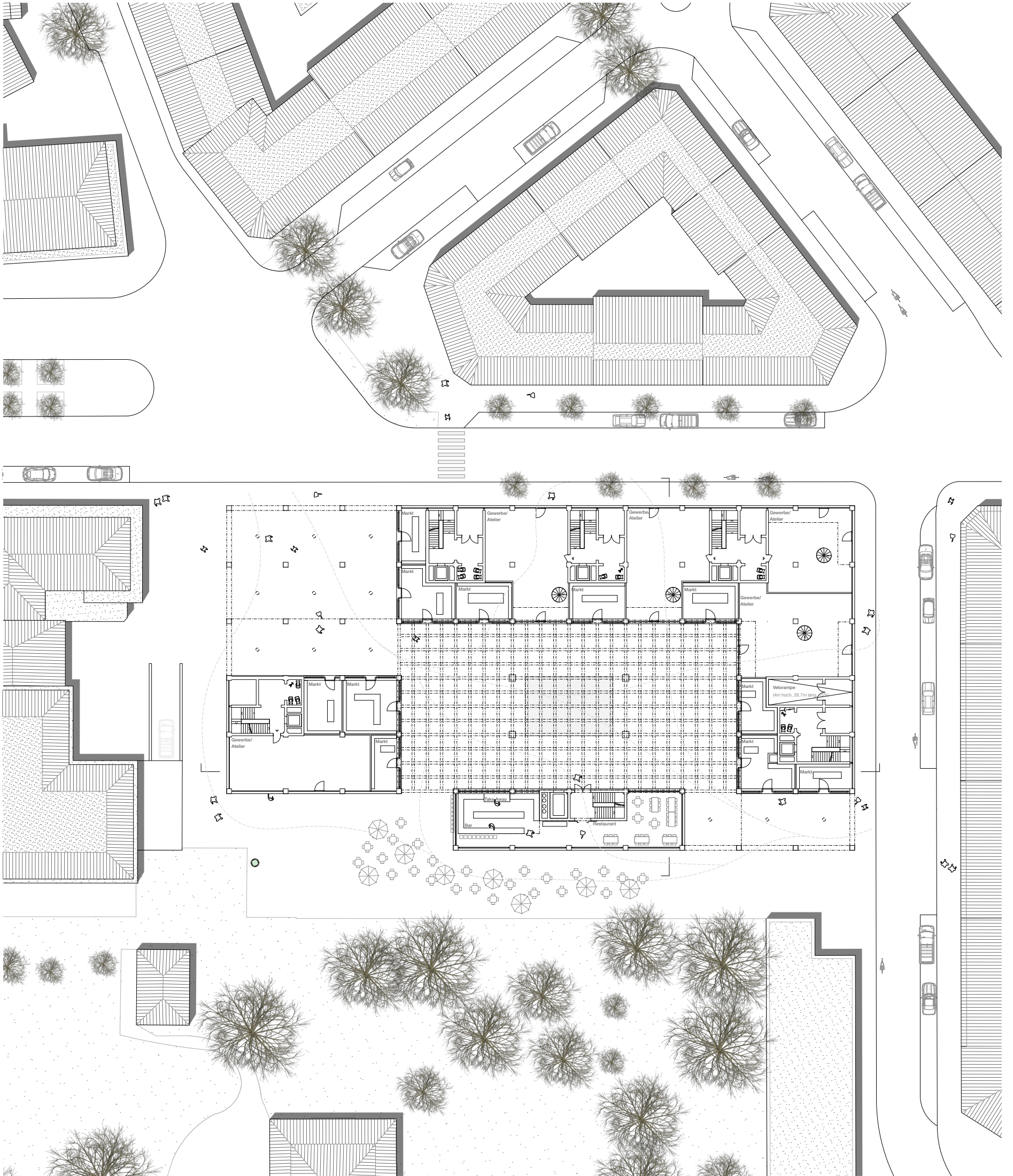
Erdgeschoss 1:500 – Markthalle, Gewerbe und Gebäudezugänge
