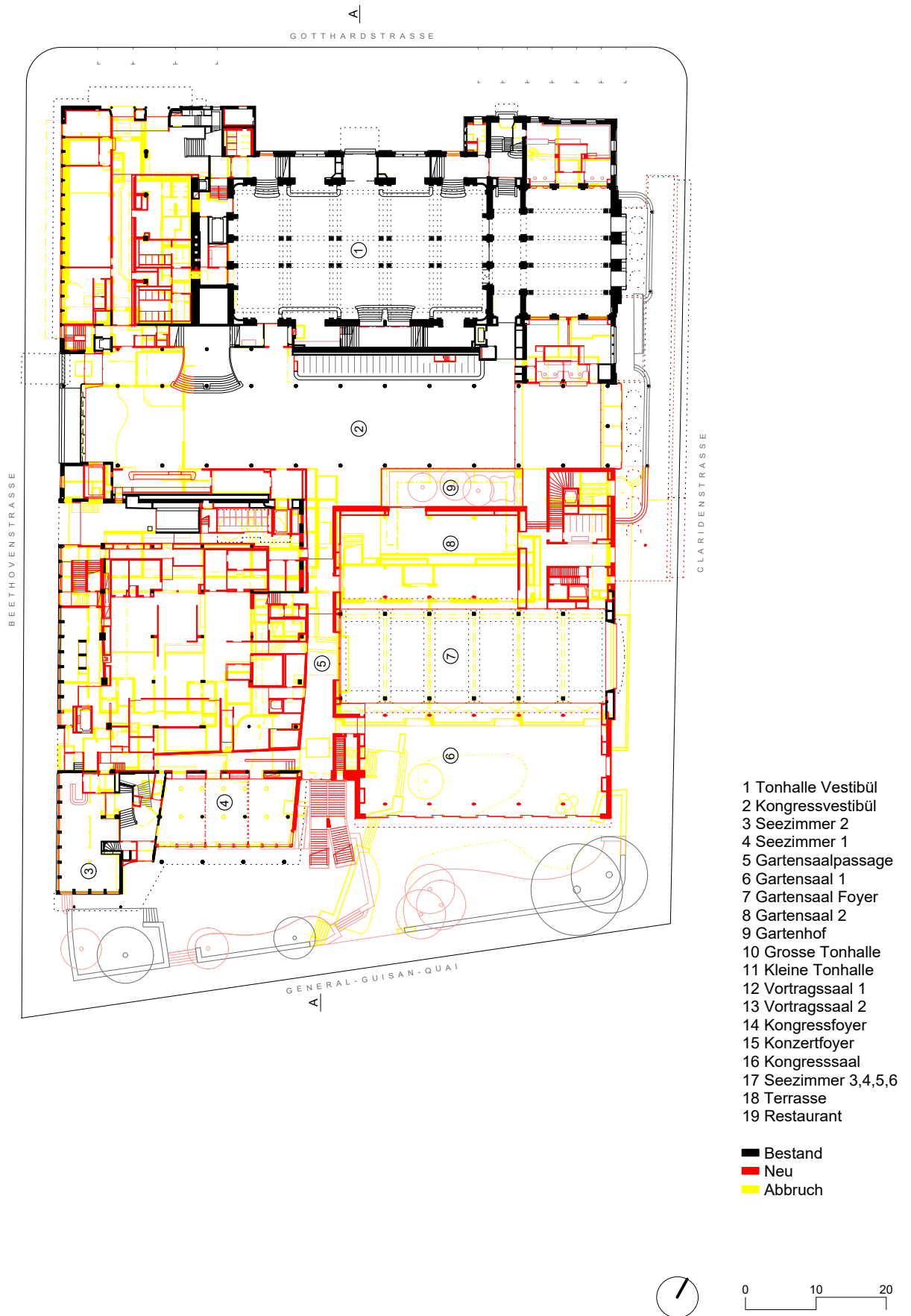
Publikationsplan, Kongresshaus / Tonhalle (VORABZUG) Grundriss Erdgeschoss, 1:800 / A4 ARGE Boesch Diener
