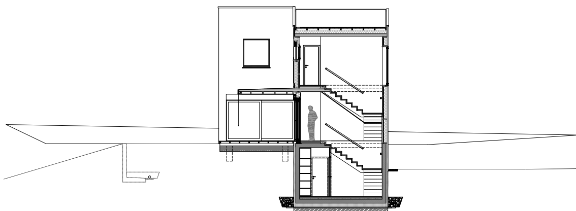
COUPE TRANSVERSALE
