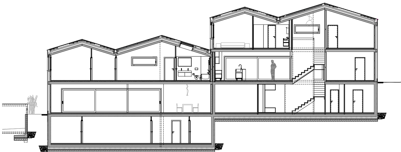
COUPE LONGITUDINALE
