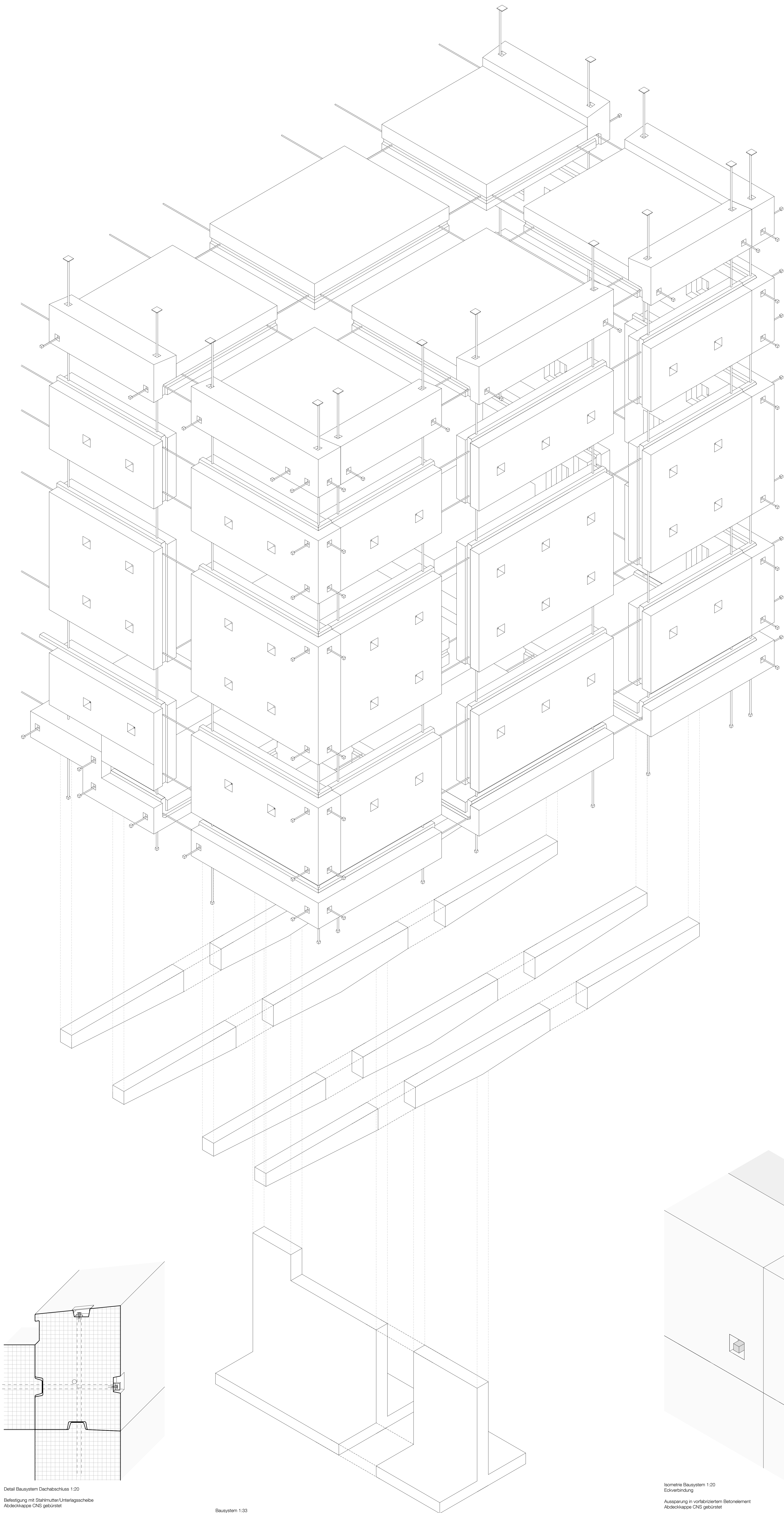
Bausystem 1:33
