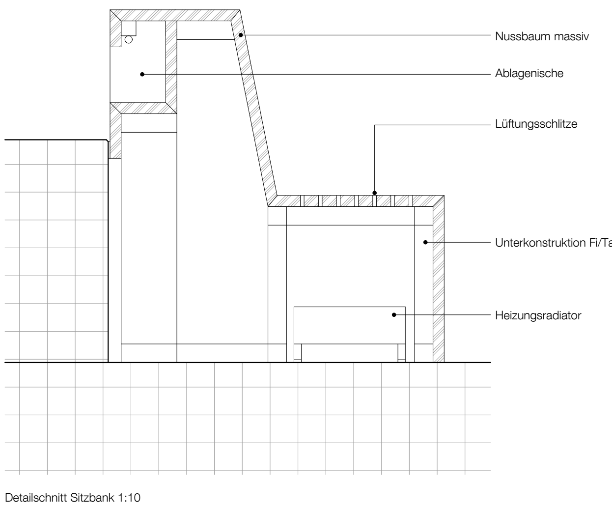
Detailschnitt Sitzbank 1:10
