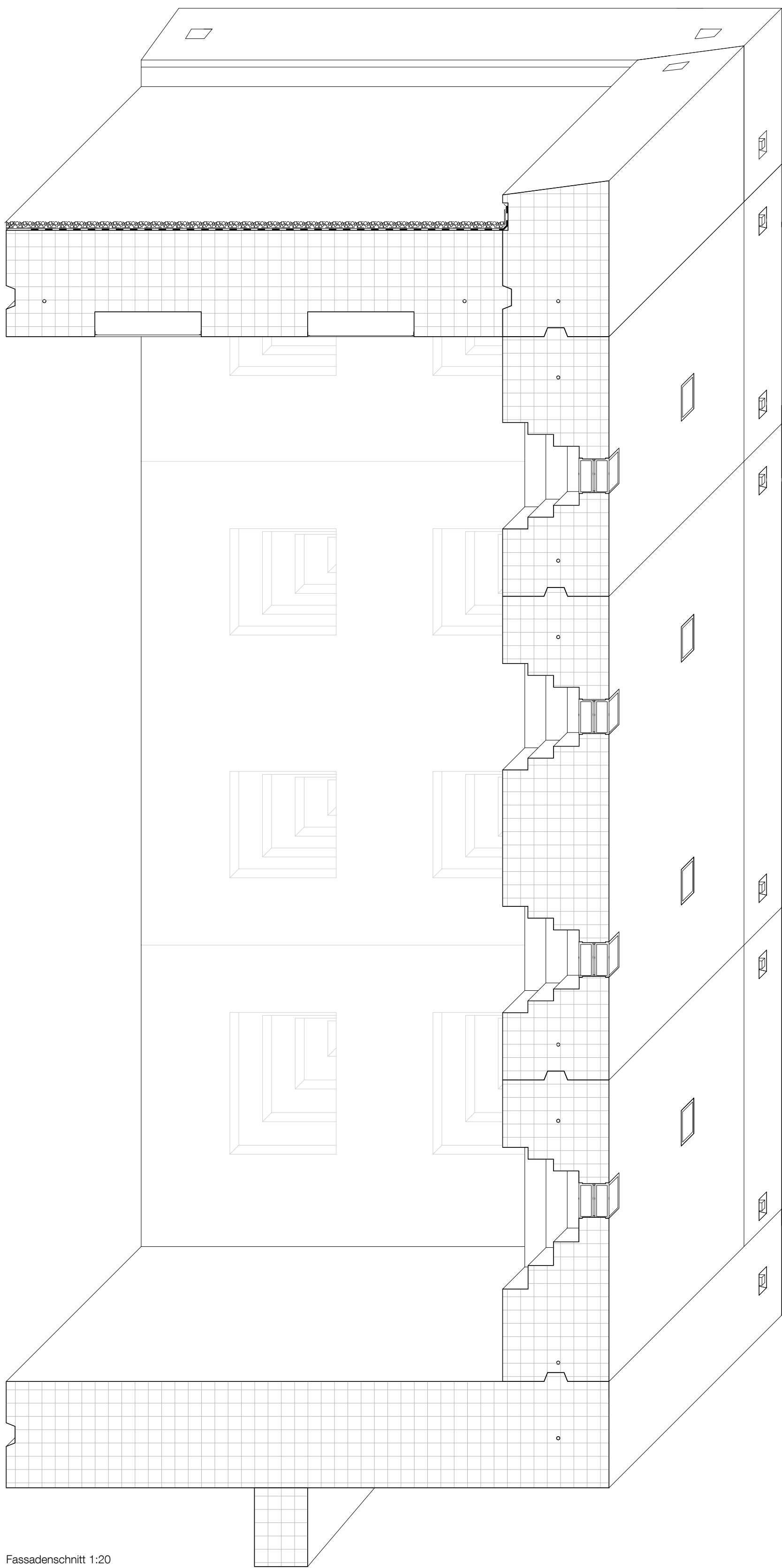
Fassadenschnitt 1:20
