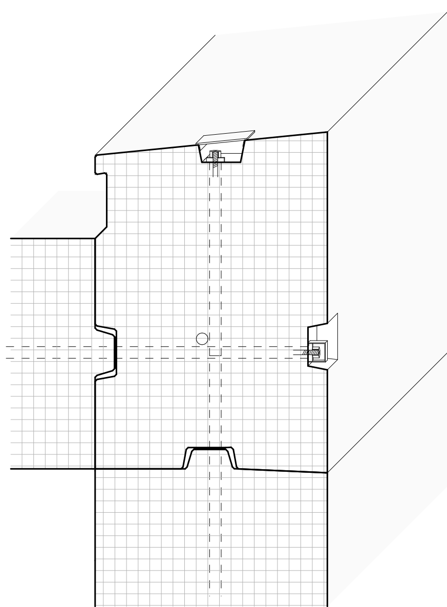
Detail Bausystem Dachabschluss 1:20 Befestigung mit Stahlmutter/Unterlagsscheibe Abdeckkappe GNS gebürstet
