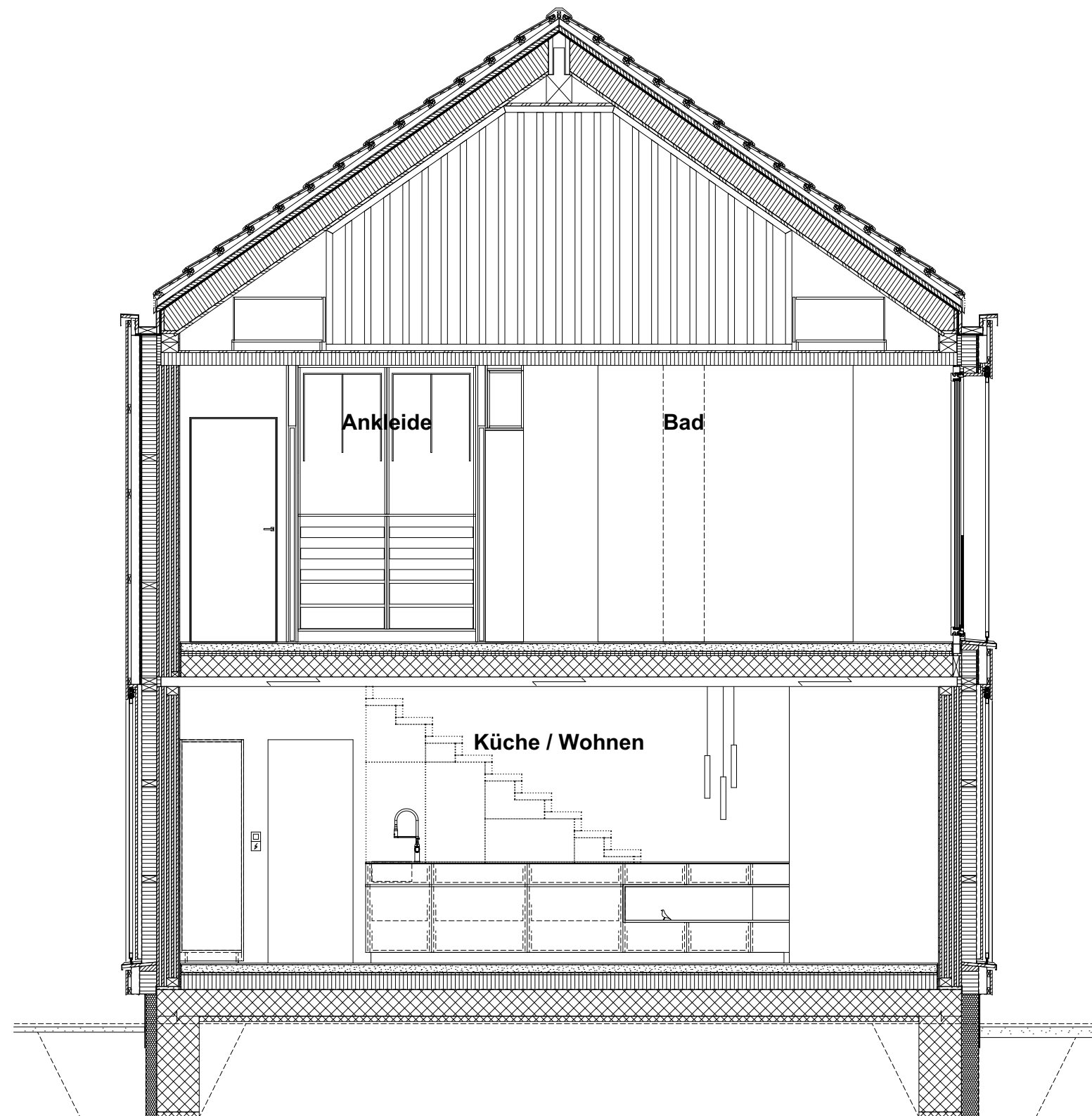
Querschnitt
