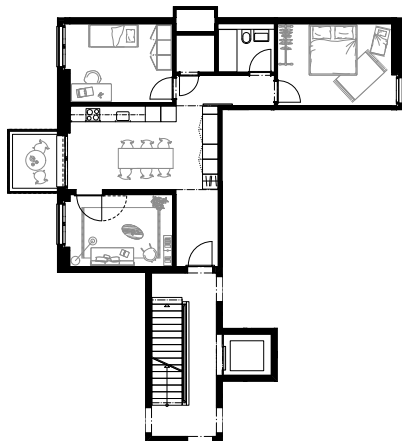
3-Zimmerwohnung
