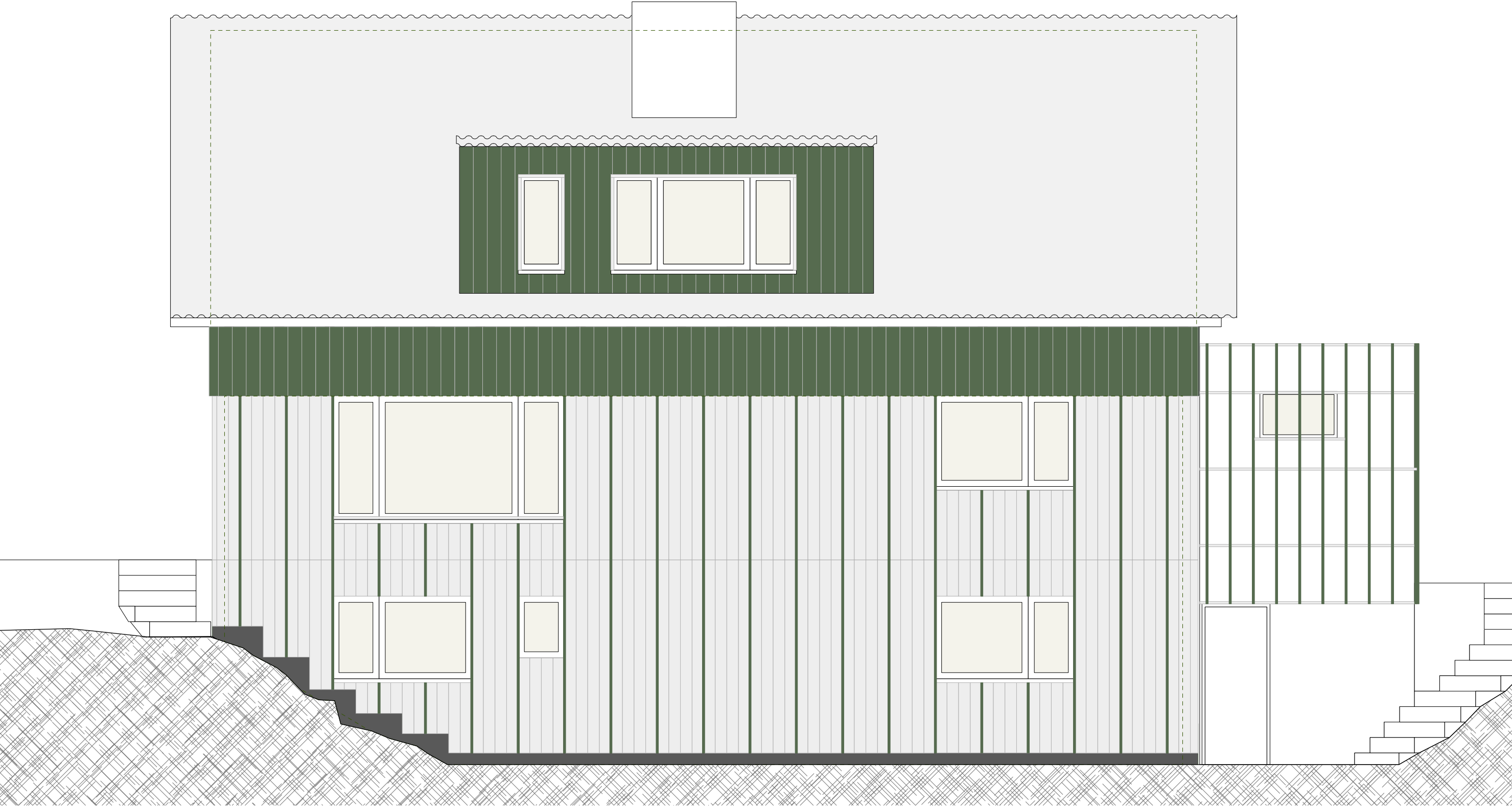
Ansicht Nord
