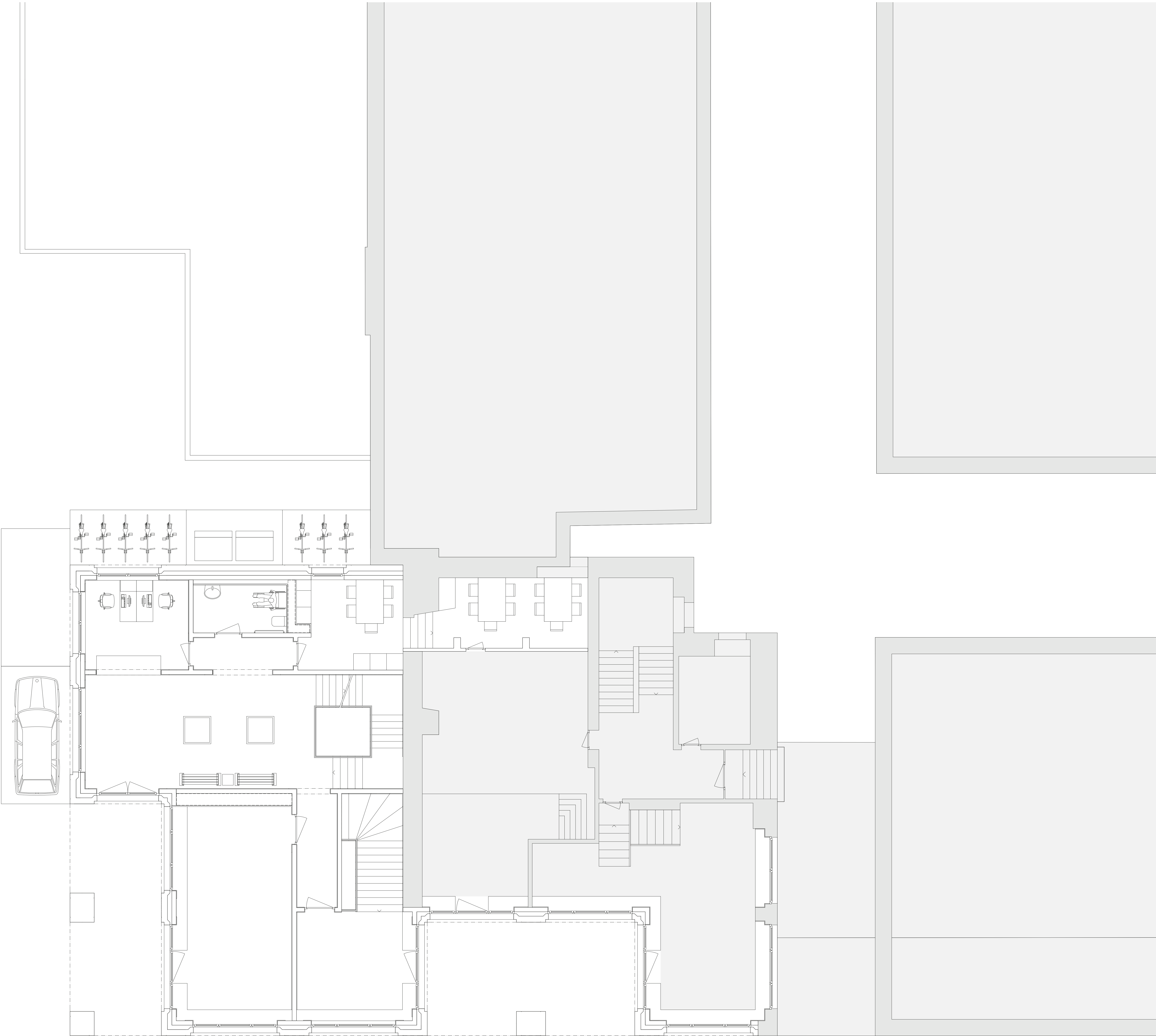
Grundriss Erdgeschoss 1:50
