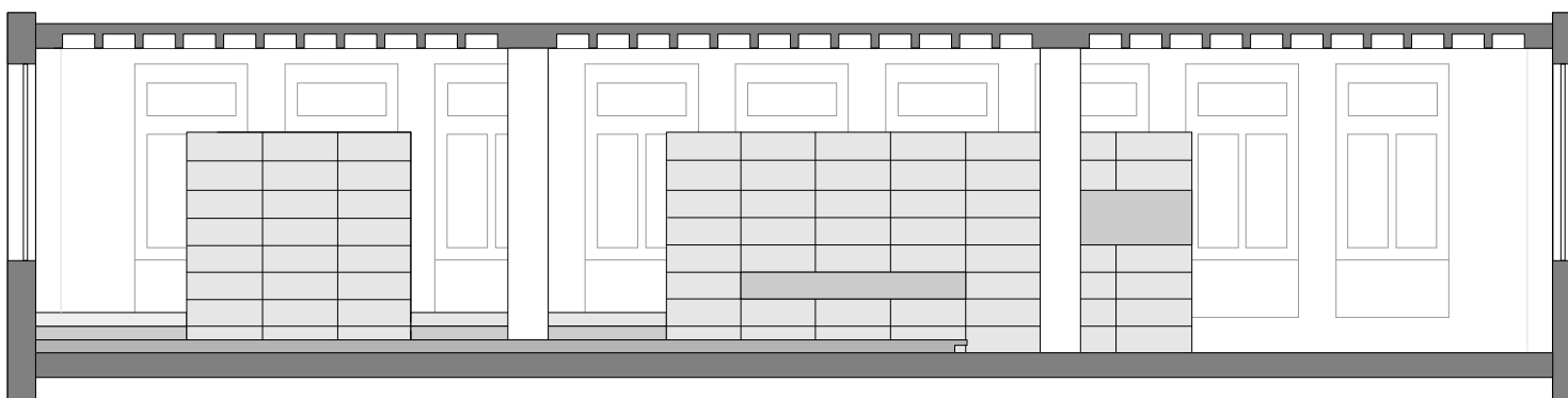
coupe longitudinale
