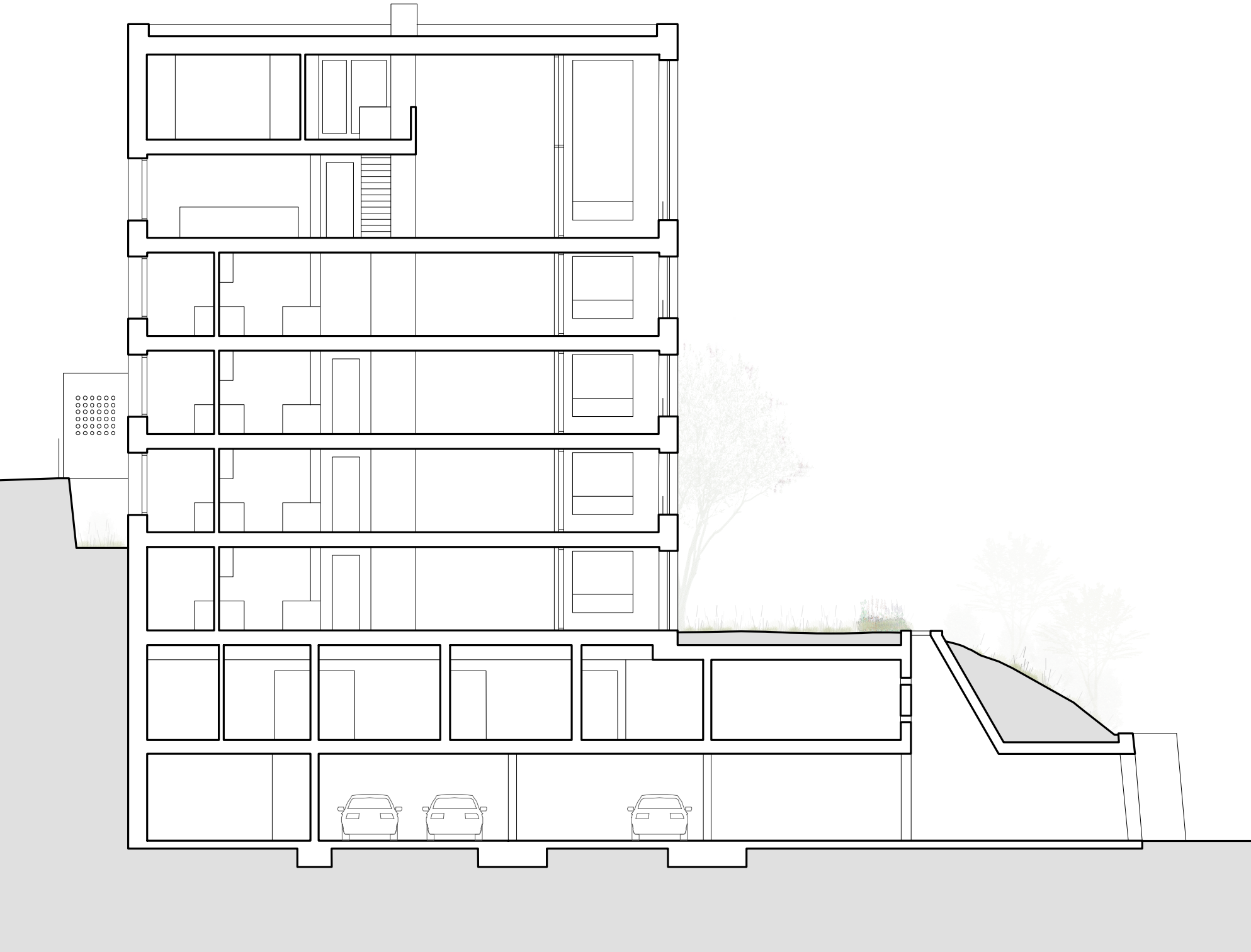
Schnitt A-A'
