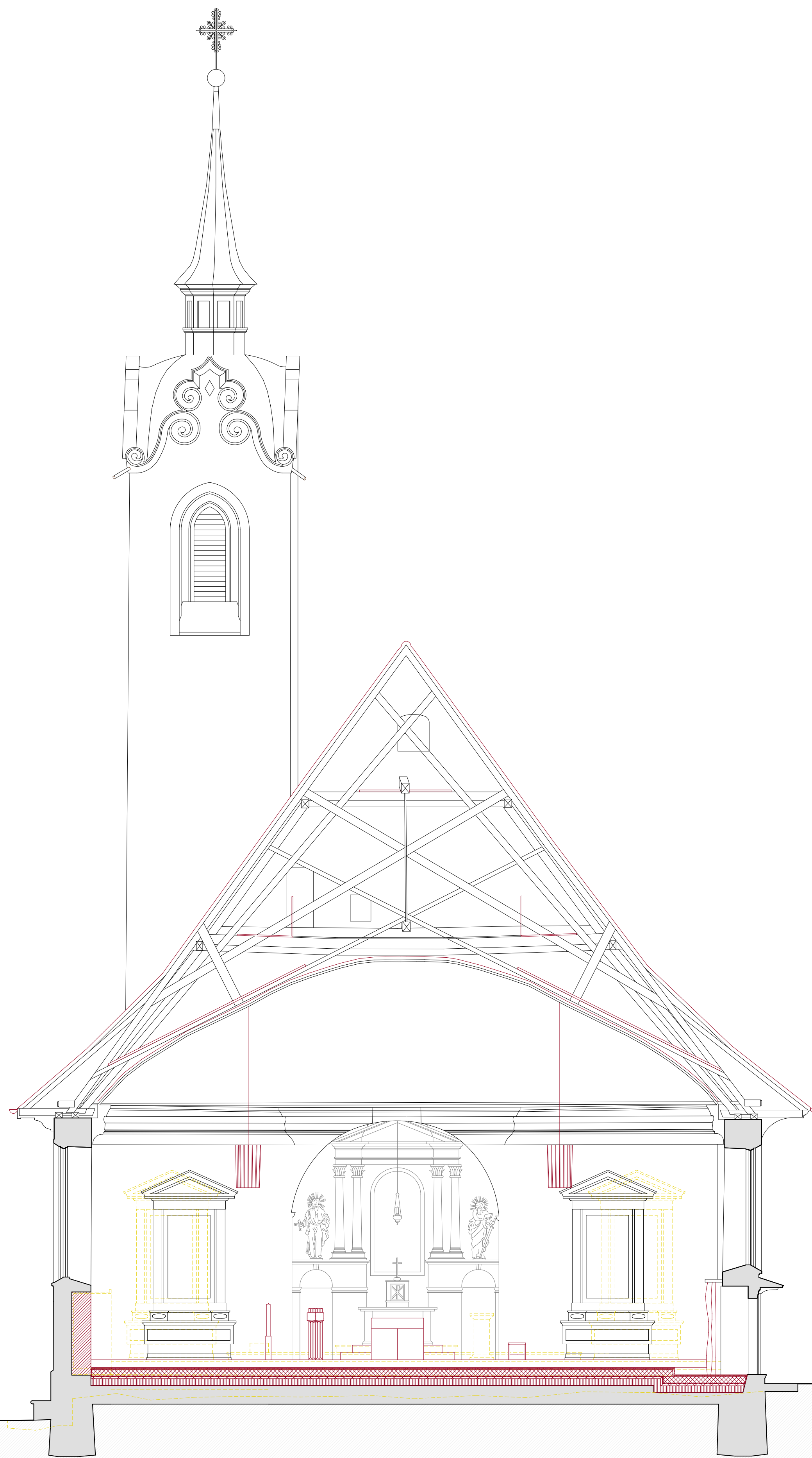
Schnitt A - A
