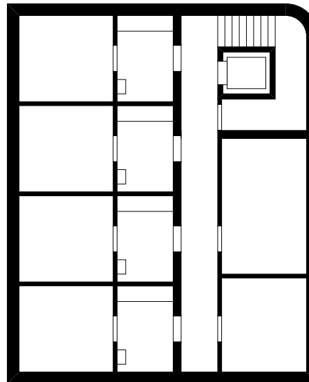
Grundriss UG
