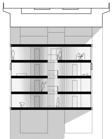
COUPE LOGEMENTS 1:200
