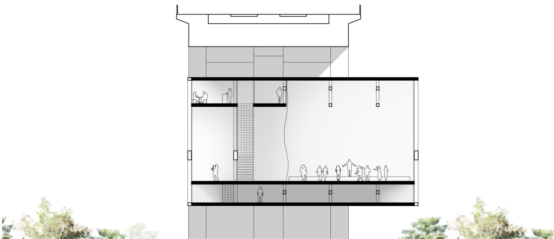
COUPE SALLE DE CONCERT 1:200
