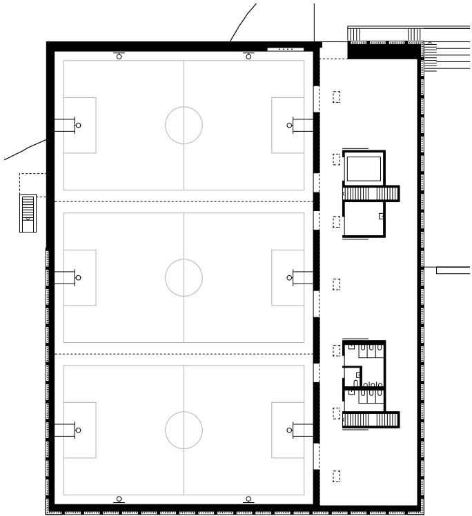
1. Obergeschoss | 1er étage
