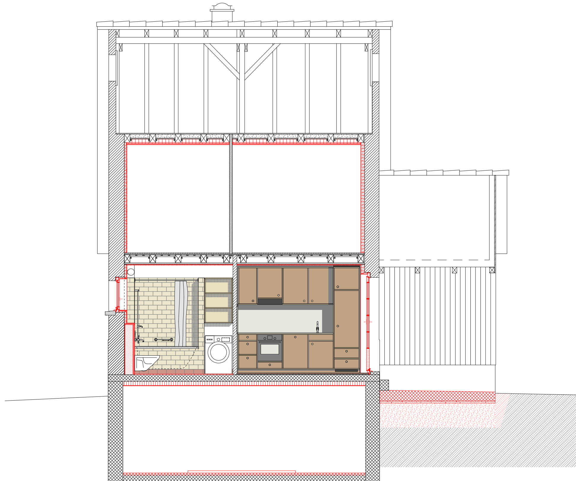
Querschnitt
