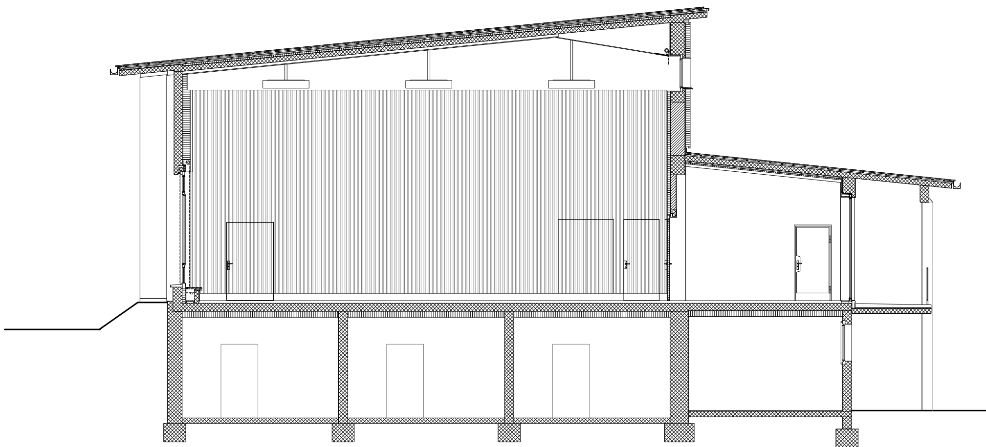
Detailschnitt Aula 0 1 2
