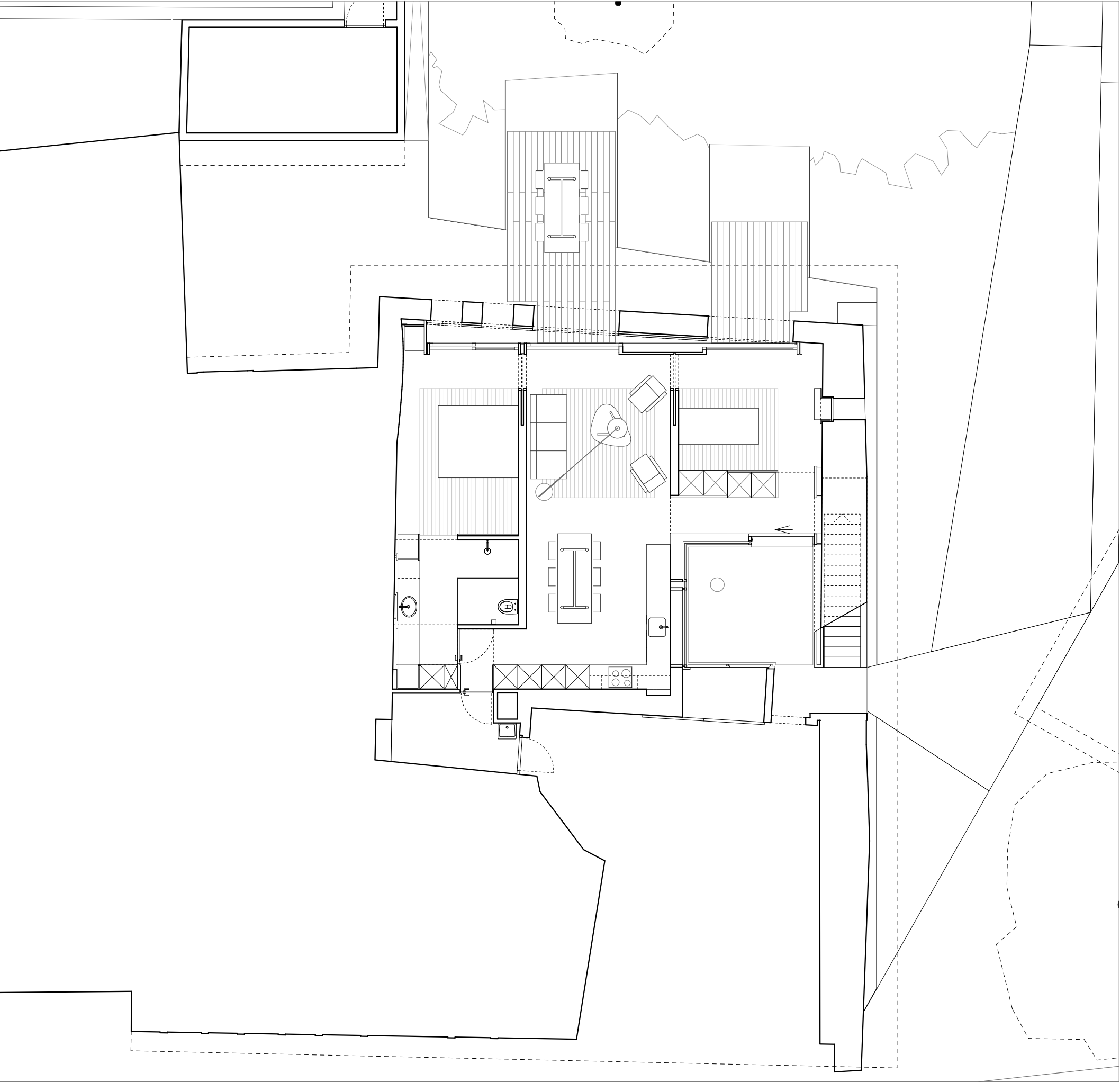
plan niveau 0
