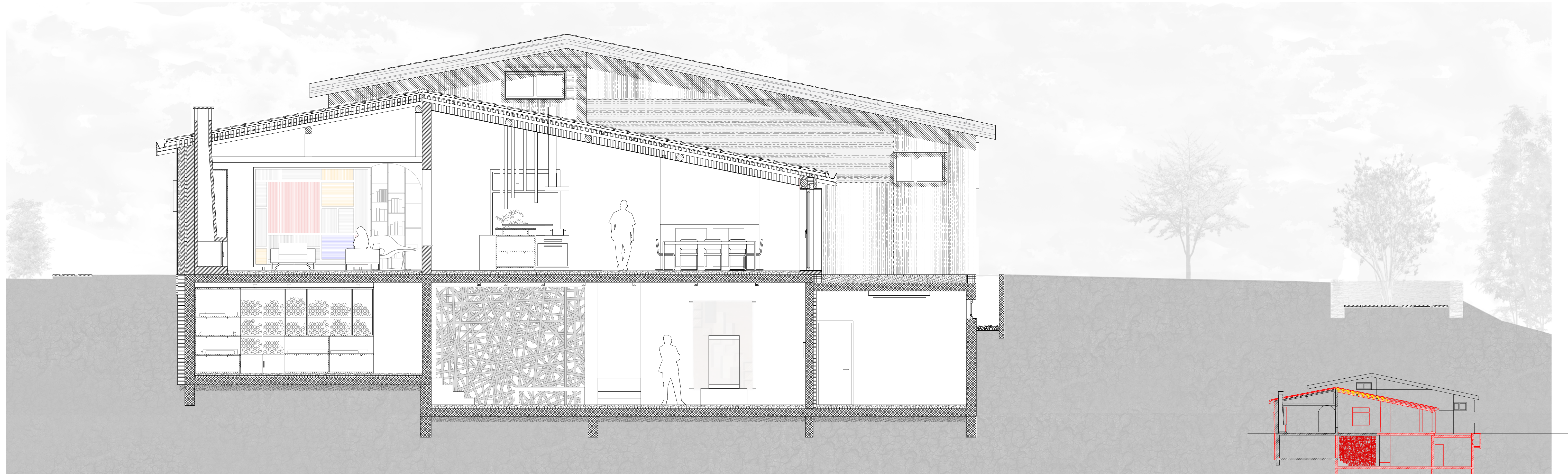
SEZIONE B-B' SCALA 1:50
