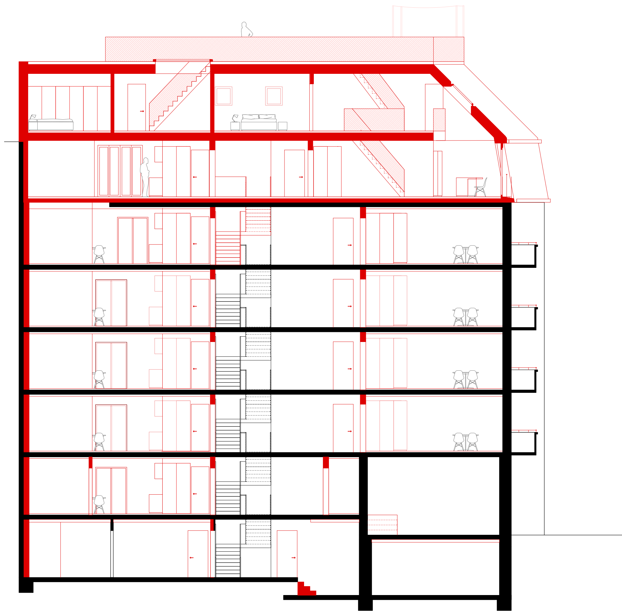
Schnitt EE
