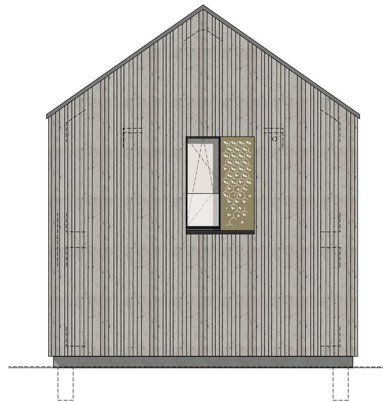
Nordfassade
