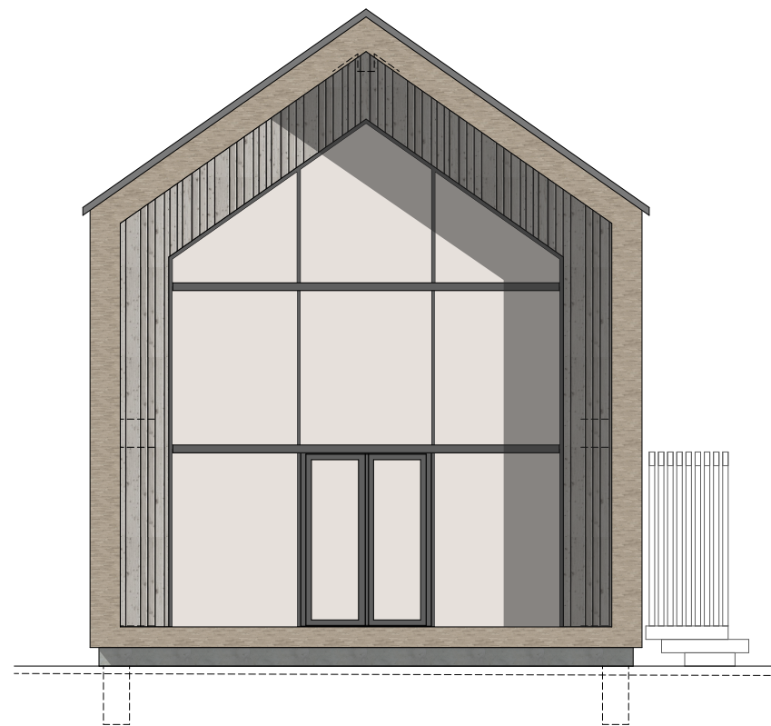
Südfassade
