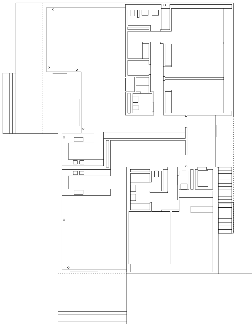
ERDEGESCHOSS
