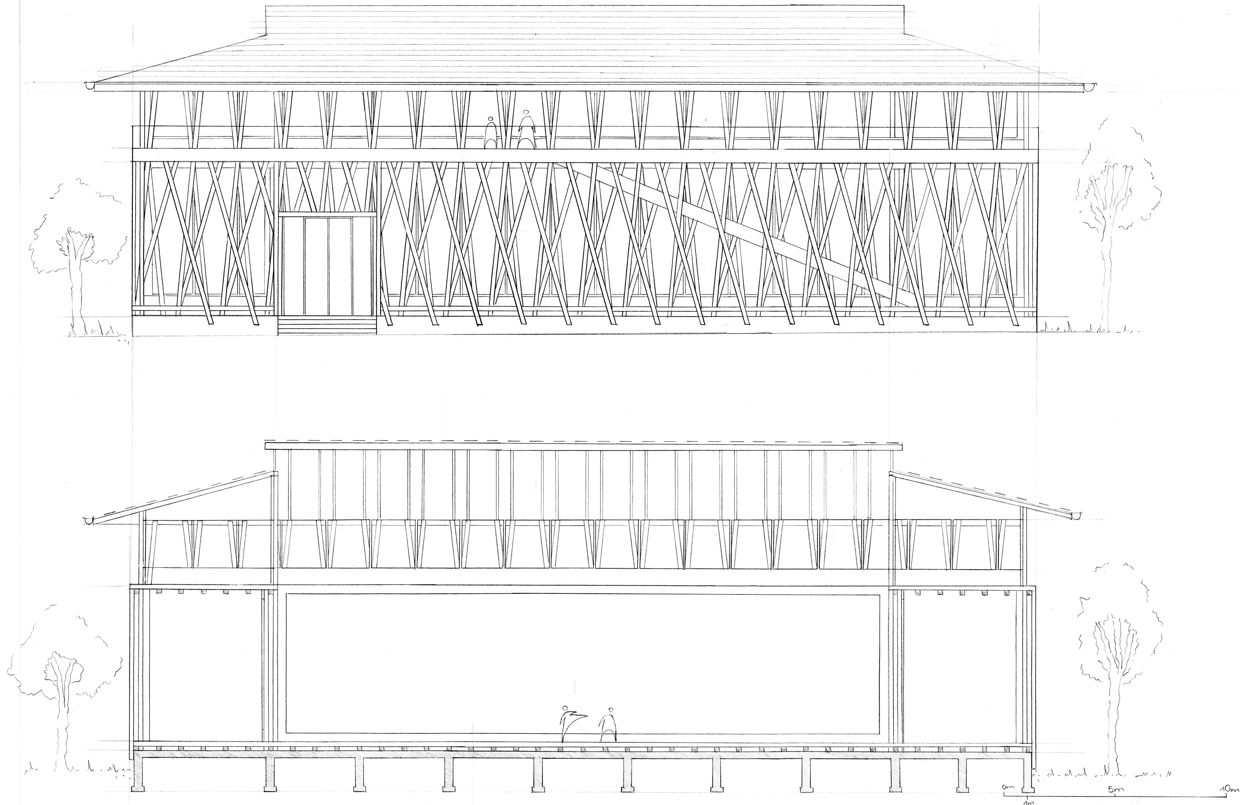
Ansicht Südost | Schnitt 1:100 Lang
