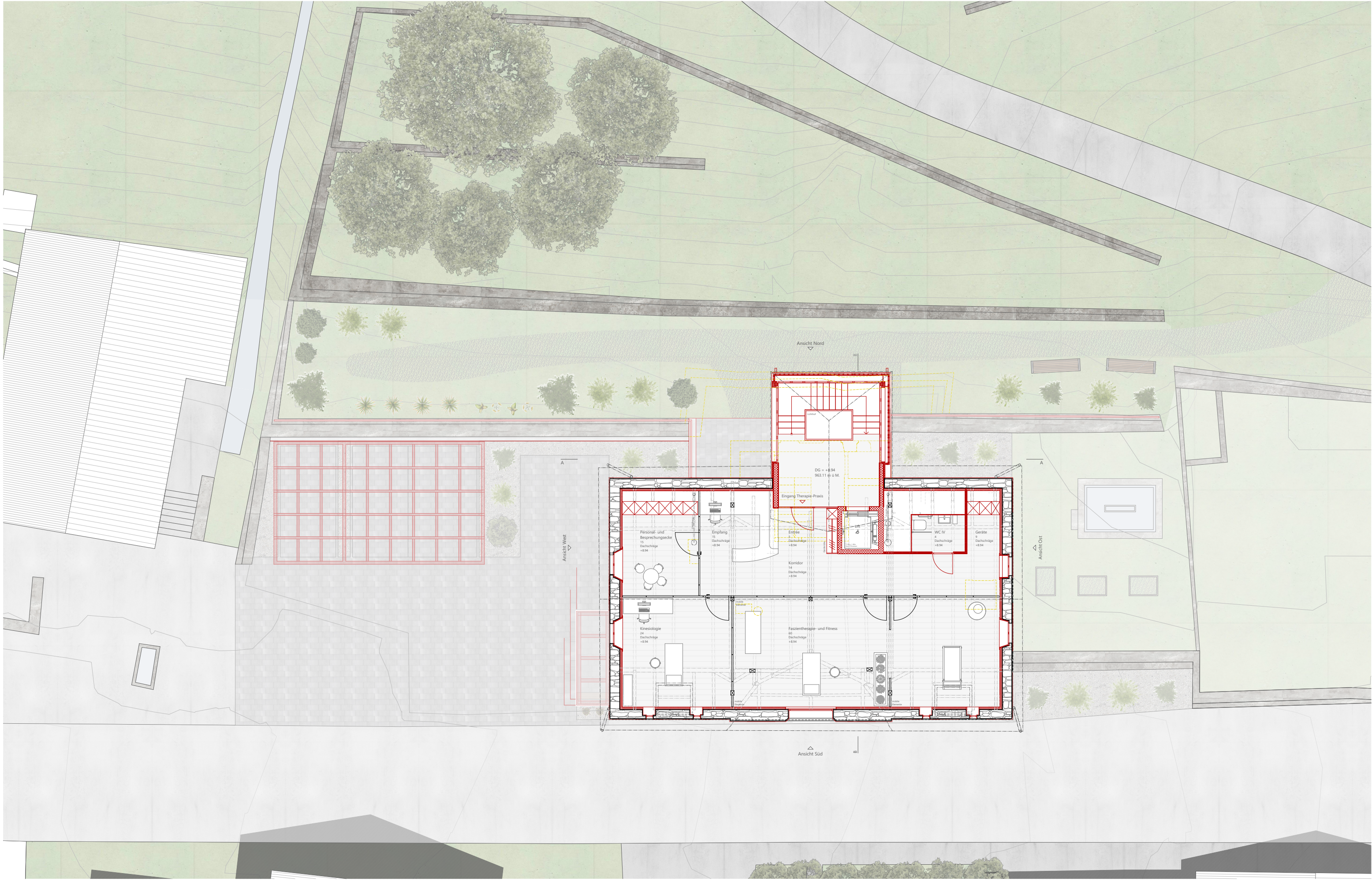
Dachgeschoss | 1:150
