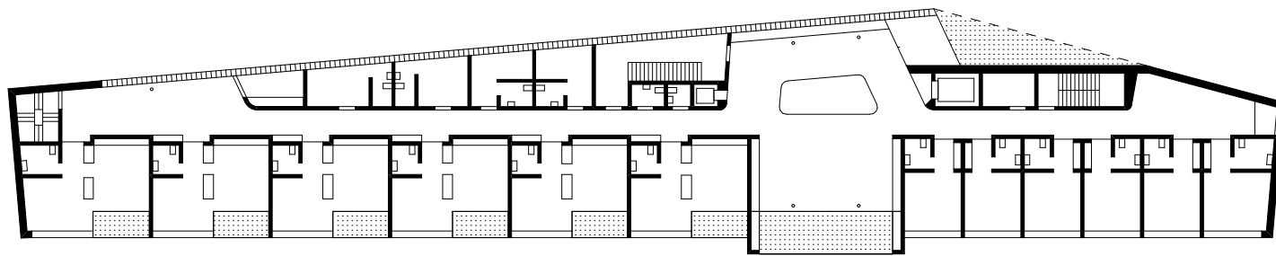
Grundriss Ebene 0
