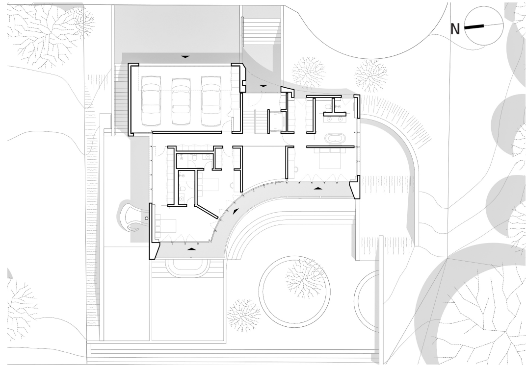
EG Grundriss
