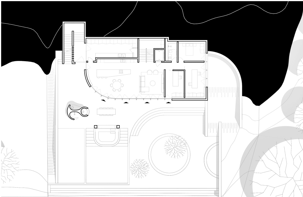
UG1 Grundriss
