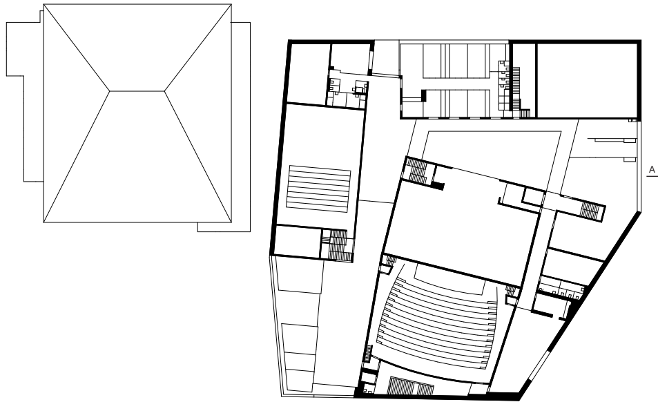
Obergeschoss | Étage
