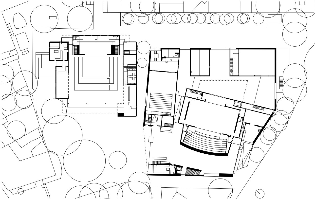
Erdgeschoss | Rez-de-chaussée
