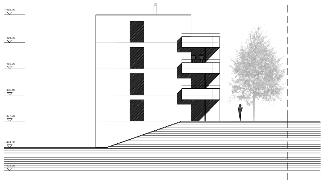
WESTFASSADE
