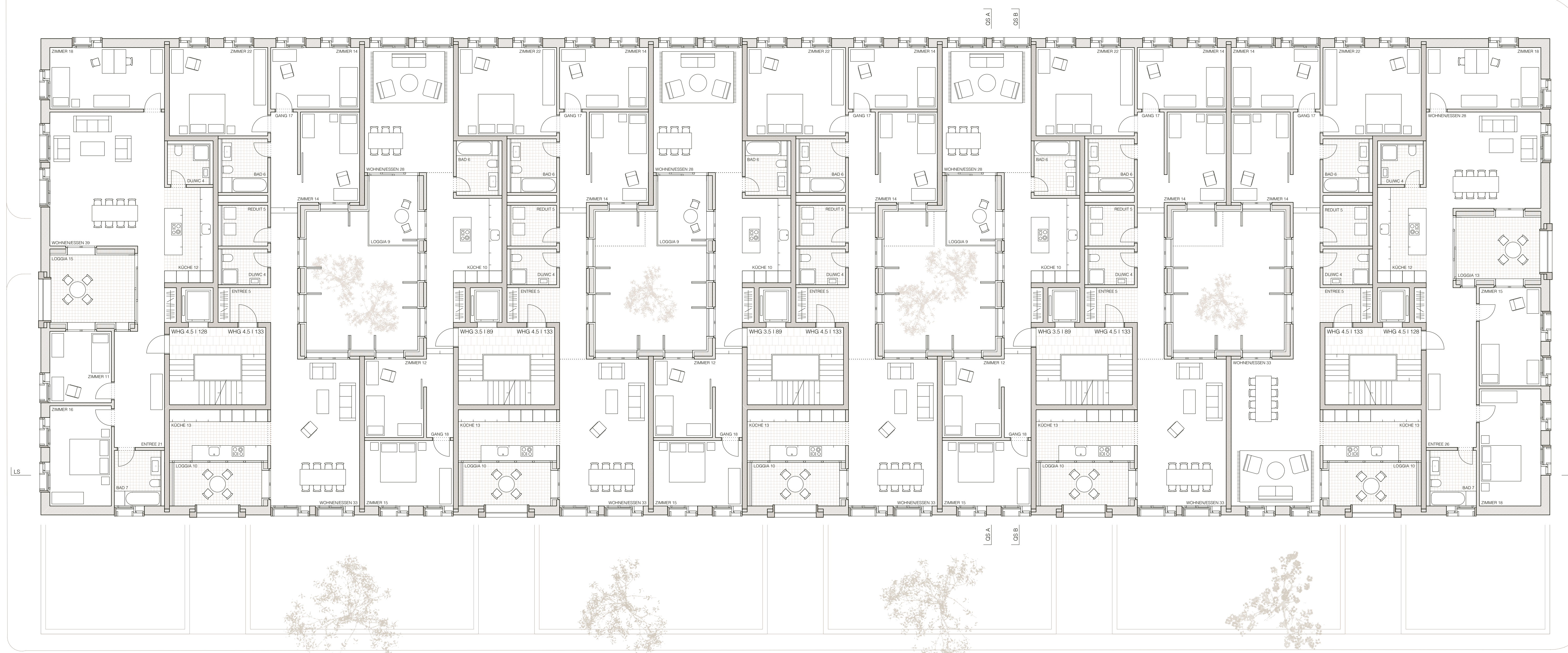
GRUNDRISS 1. OBERGESCHOSS 1:100
