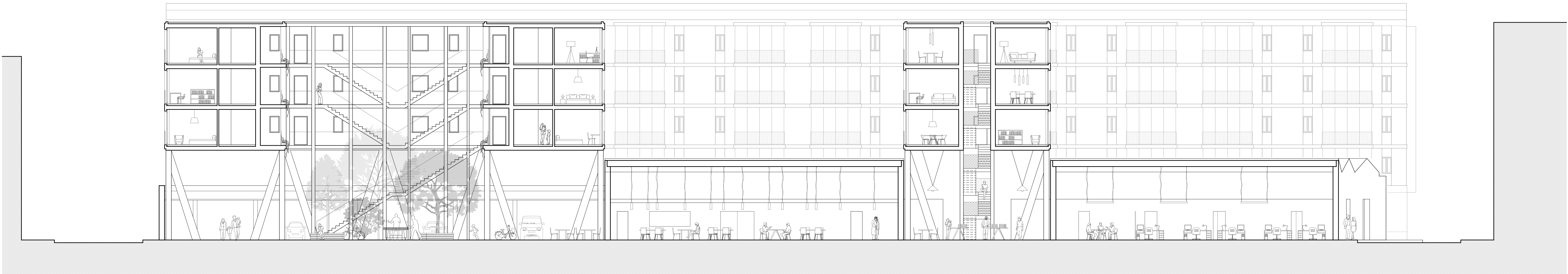
Schnitt 1:100
