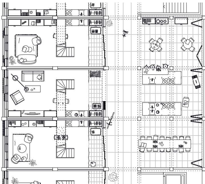
Heute 1. Etagegeschoss unten 1:50
