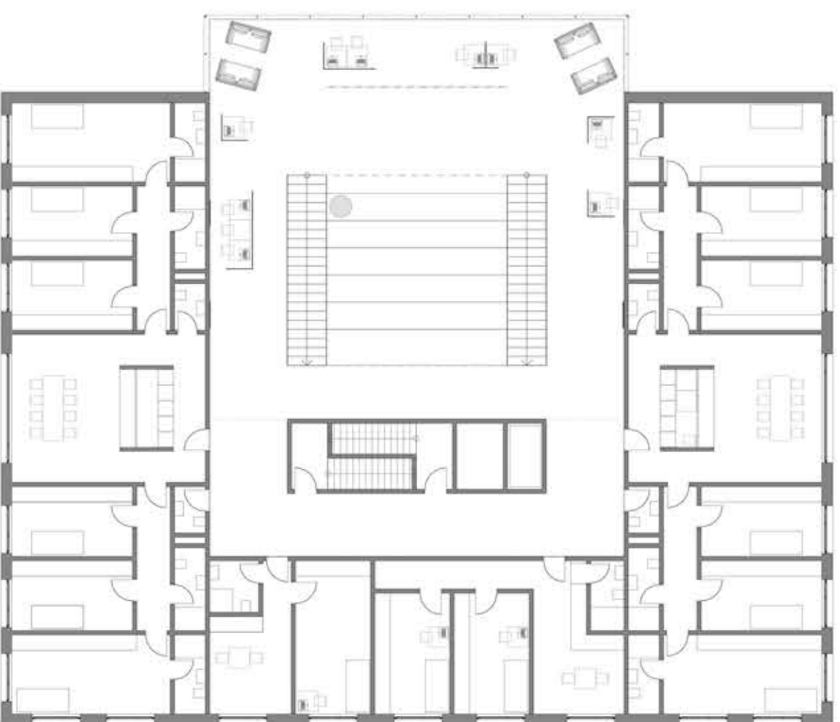
2. Obergeschoss 1:200
