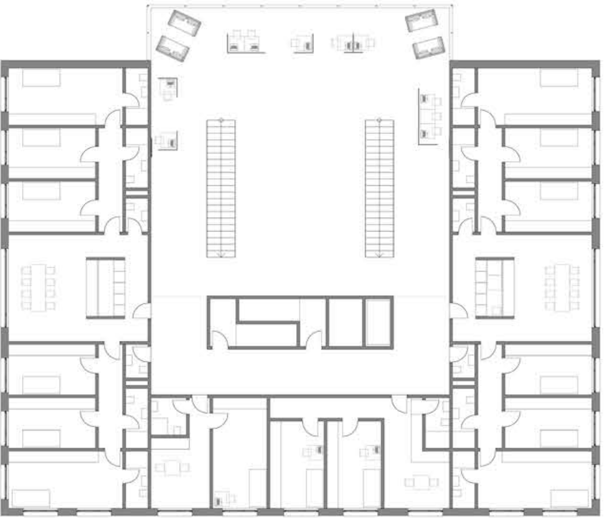
5. Obergeschoss 1:200
