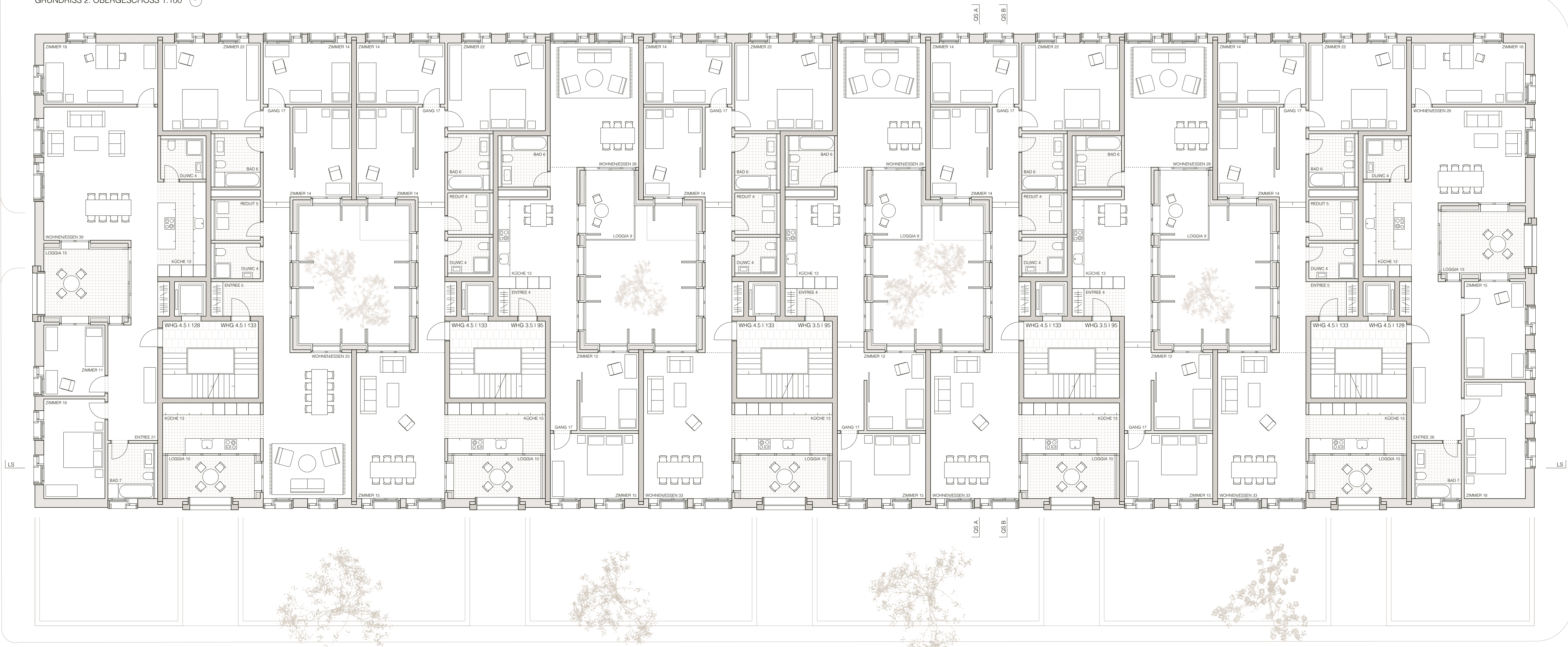
GRUNDRISS 2. OBERGESCHOSS 1:100
