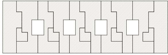
GRUNDRISS 2. OBERGESCHOSS 1:100
