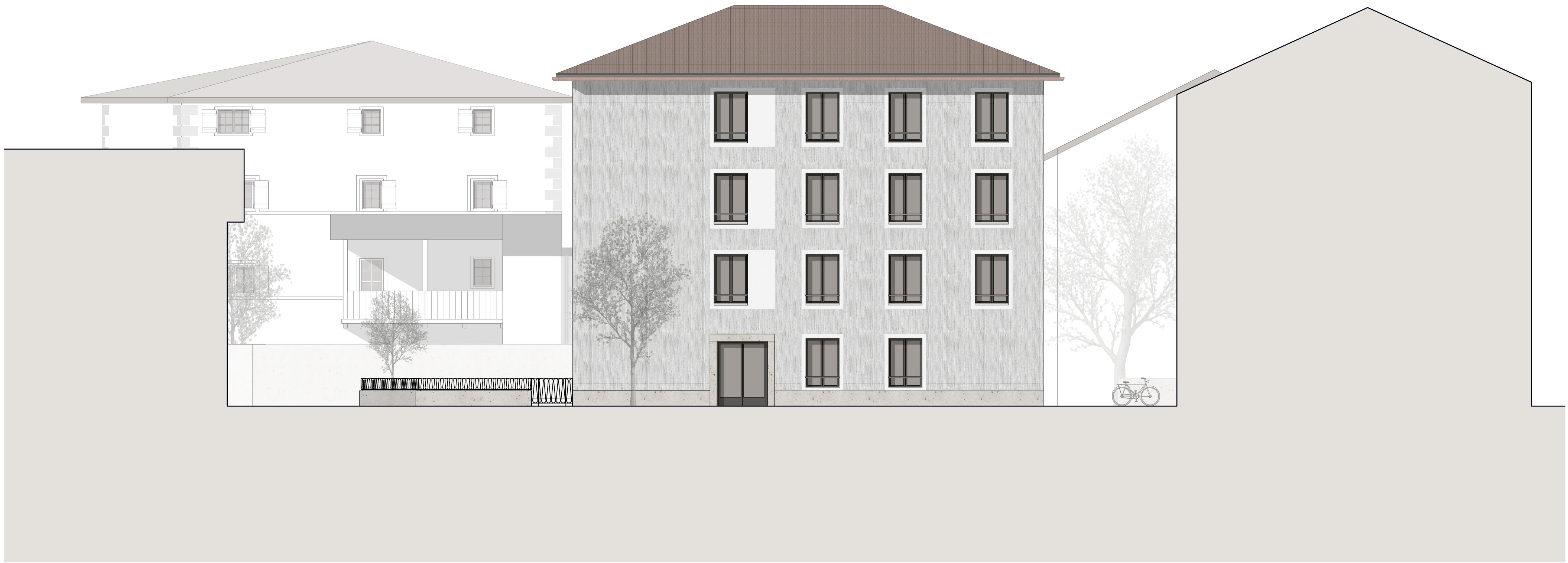
Fassadenansicht Nord-Ost | Mst. 1:100
