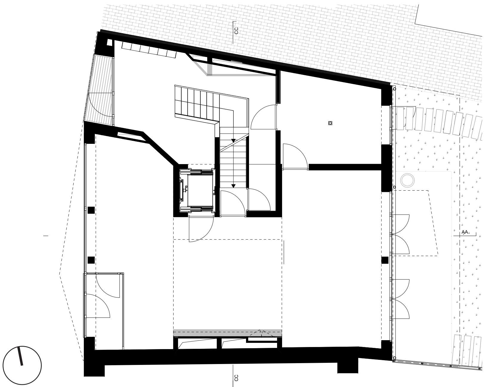
Erdgeschoss
