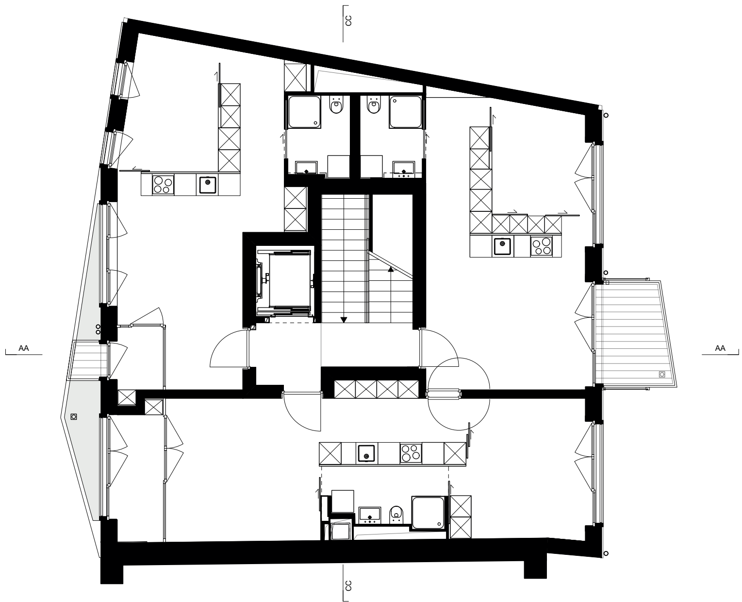
1.-3. Obergeschoss
