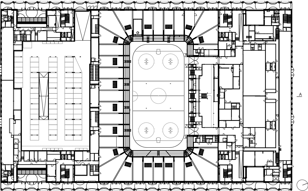
Erdgeschoss | Rez-de-chaussée
